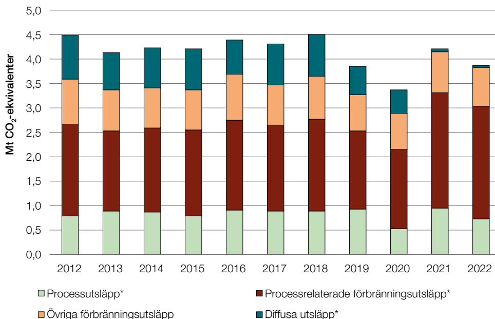
Figur 10. Raffinaderiers och kemiindustrins utsläpp av fossila växthusgaser fördelat på olika utsläppskategorier, 2012–2022, miljoner ton koldioxidekvivalenter (kategorier markerade med * ingår i processrelaterade utsläpp).
