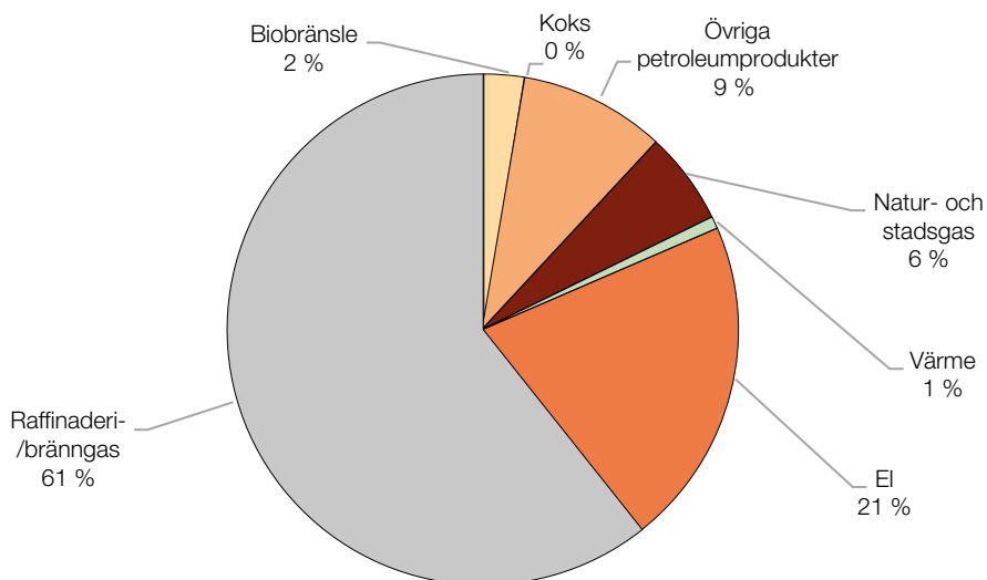
Figur 11. Raffinaderiers och kemiindustrins (inklusive läkemedelsindustrins) energianvändning fördelat på olika energikällor, 2022, procent.
