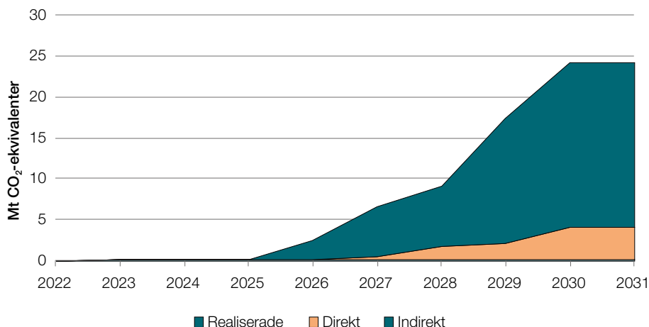
Figur 5. Utsläppsminskningspotential för projekt som stöds av Industrikivet fördelat på realiserade, direkta och indirekta utsläpp (baserat på företagens egna uppgifter), i miljoner ton koldioxidekvivalenter.
