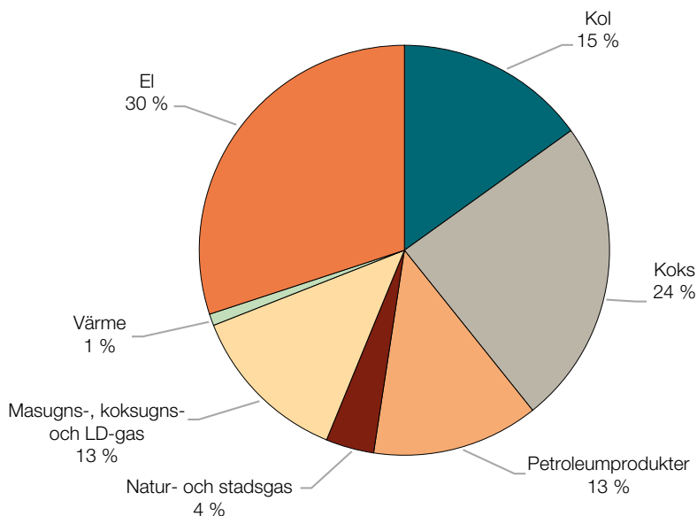
Figur 9. Järn- och stålindustrins energianvändning, inklusive järnmalmshugvuror och koksverk, fördelat på olika energikällor, 2022, procent.
