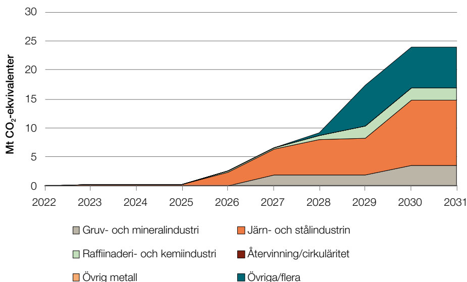
Figur 6. Utsläppsminskningspotential per bransch och år för projekt som stöds av Industrikivet (baserat på företagens egna uppgifter), i miljoner ton koldioxidekvivalenter.
