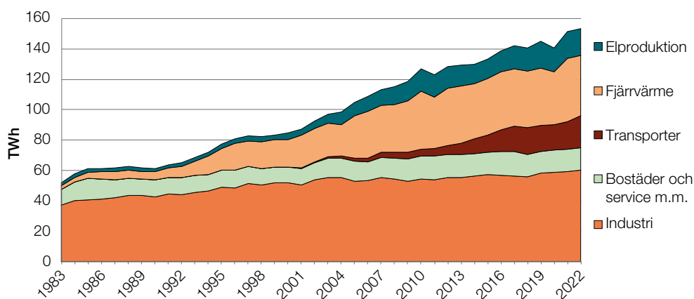
Figur 16. Användning av biobränsle per sektor, 1990–2022, TWh.
