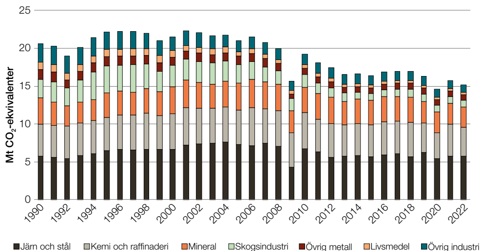
Figur 3. Industrins totala utsläpp av fossila växthusgaser fördelat på olika branscher, 1990–2022, miljoner ton koldioxidekvivalenter.
