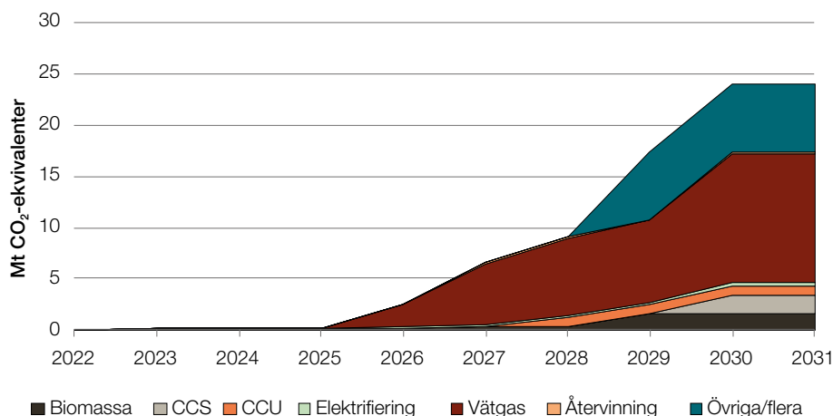
Figur 7. Utsläppsminskningspotential per teknikspår och år för projekt som stöds av Industriklivet (baserat på företagens egna uppgifter), i miljoner ton koldioxidekvivalenter.
