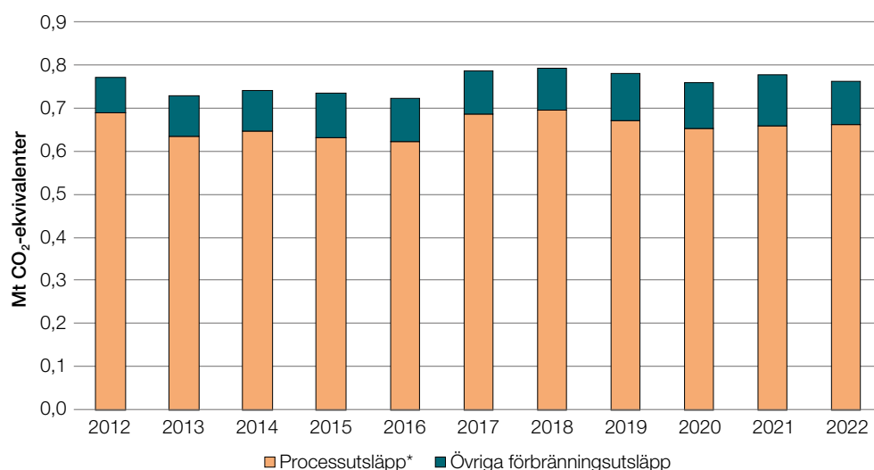
Figur 14. Övrig metallindustris utsläpp av fossila växthusgaser fördelat på olika utsläppskategorier, miljoner ton koldioxidekvivalenter, 2012–2022 (kategorier markerade med * ingår i processrelaterade utsläpp).
