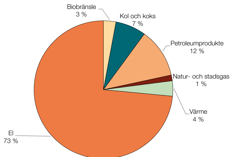
Figur 15. Energianvändningen i övrig metallindustri fördelat på olika energikällor, 2022, procent.
