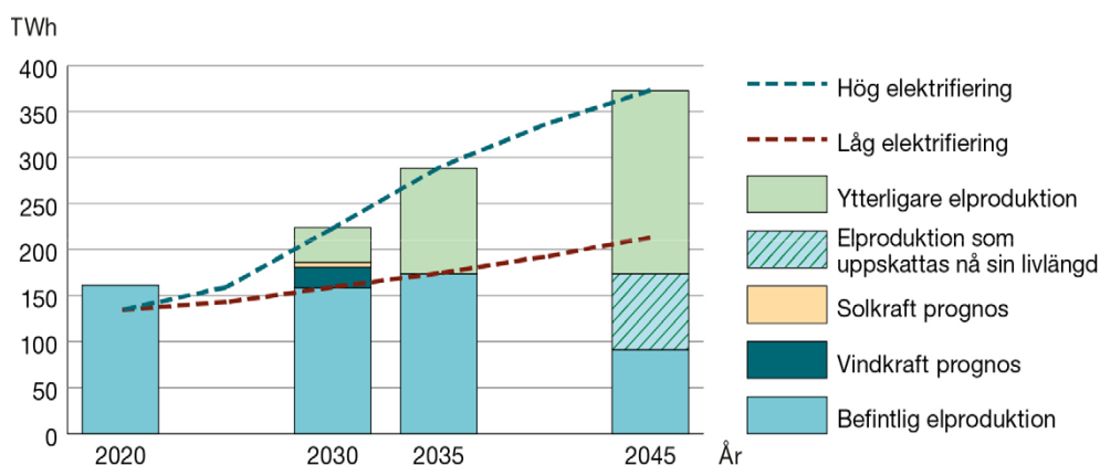
Figur 3: Ökning av elbehovet till 2045 (utfallsrummet mellan de streckade linjerna, se kapitel 2) i jämförelse med befintlig elproduktion, prognoser över tillskott och ytterligare behov för att nå de högre utfallet.
