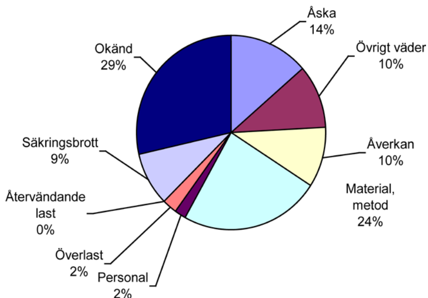
Figur 4. Avbrottsorsaker i lokalnätet (dvs. spänningsnivåer mellan 0,4–24 kV). Källa: Svensk Energis avbrottsstatistik för 2009 avseende elavbrott längre än tre minuter.
