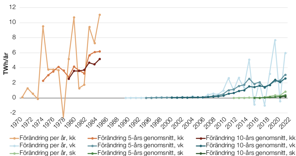
Figur 8. Utbyggnadstakt (inkl. årsvariationer) för kärnkraft (kk), vindkraft (vk) och solkraft (sk), 1970–2021, TWh/år.
