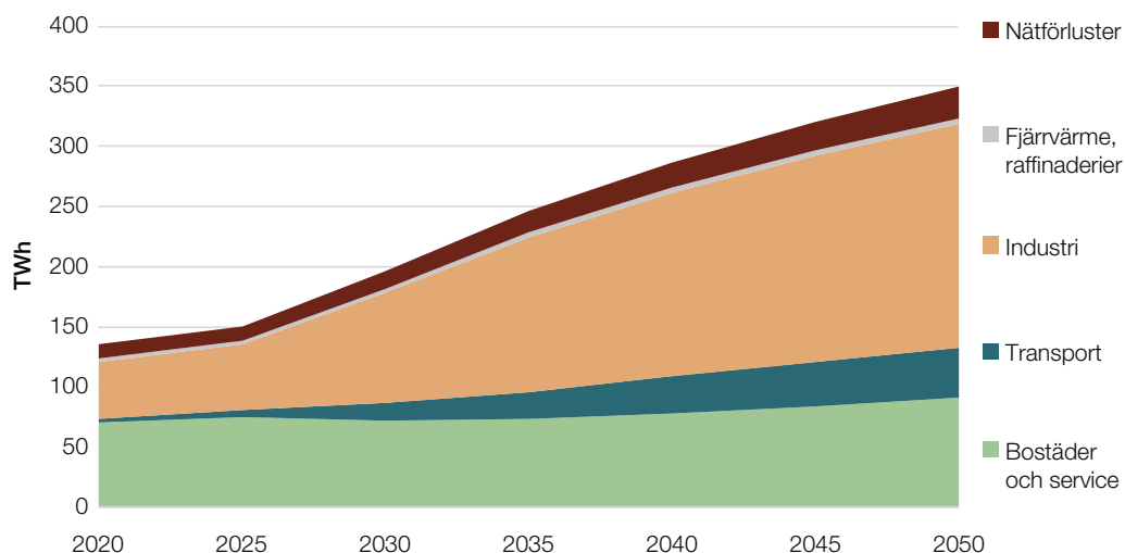
Figur 3. Elanvändning uppdelat per sektor 2020 samt 2025–2050 i scenario Högre elektrifiering, TWh.
