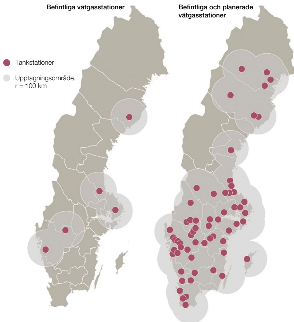
Figur 11. Befintliga och planerade vätgastankstationer, juni 2023.
