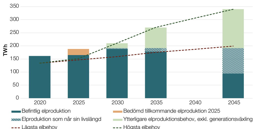
Figur 2. Bedömt ökat elbehov i kortsiktiga analyser och långsiktiga scenarier till 2045 (utfallsrummet mellan streckade linjer) jämfört med befintlig elproduktion, prognostiserat tillskott till 2025, elproduktion som når sin livslängd och ytterligare behov av elproduktion för att nå det högre elbehovet, TWh.
