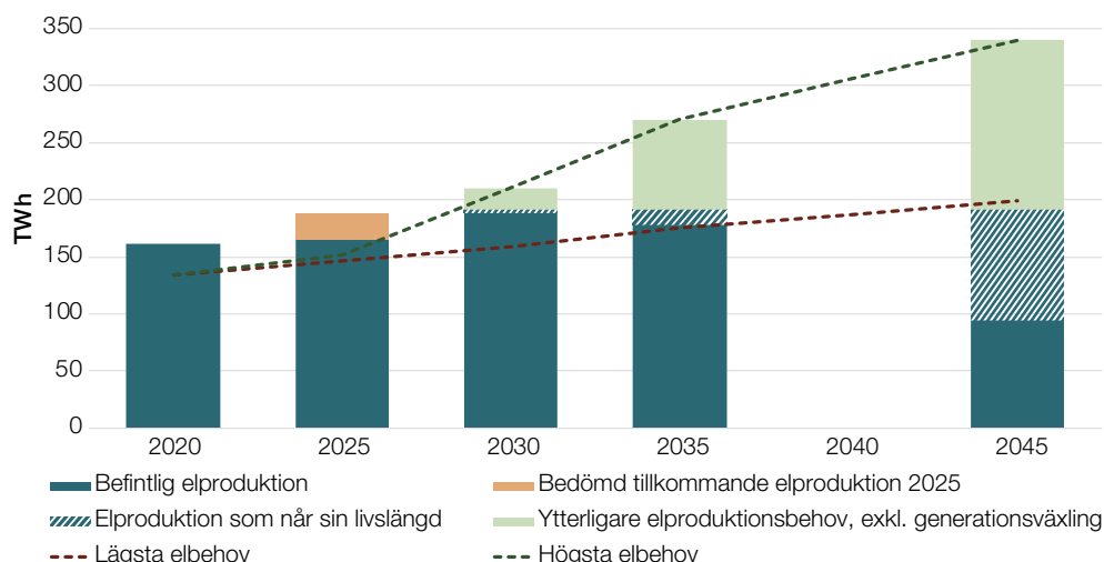
Figur 1. Bedömt ökat elbehov i kortsiktiga analyser och långsiktiga scenarier till 2045 (utfallsrummet mellan streckade linjer) jämfört med befintlig elproduktion, prognostiserat tillskott till 2025, elproduktion som når sin livslängd och ytterligare behov av elproduktion för att nå det högre elbehovet, TWh.
