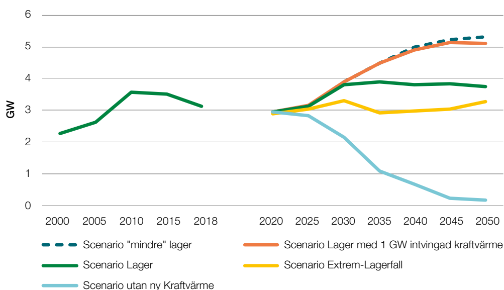
Figur 5. Installerad effekt i kraftvärmen (i fjärrvärmenäten), referensfall och olika scenarier.
