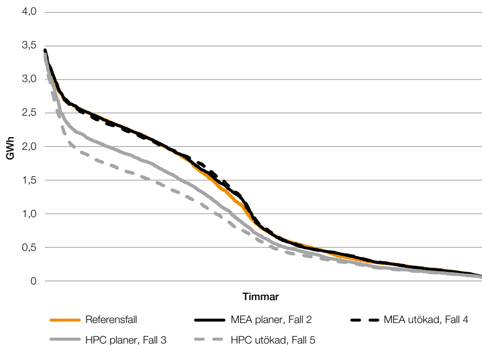
Figur 38. Varaktighet för elproduktionen från kraftvärmeverken för de olika fallen.
