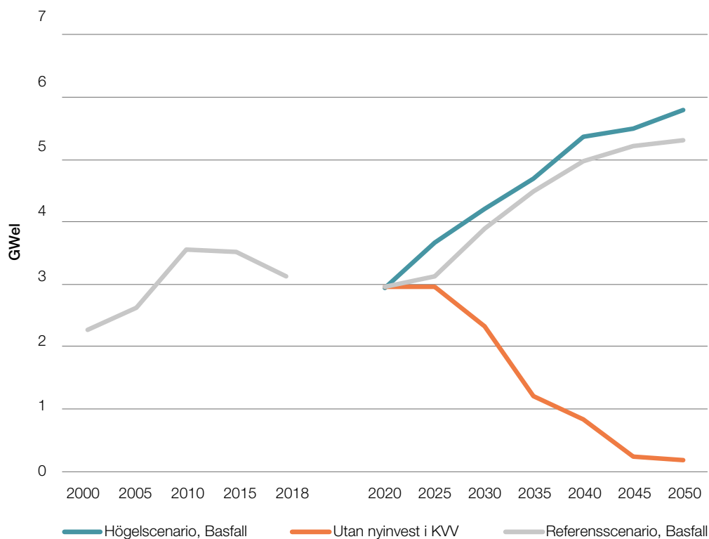
Figur 4. Installerad kraftvärmekapacitet (GWel) i de olika beräkningsfallen.
