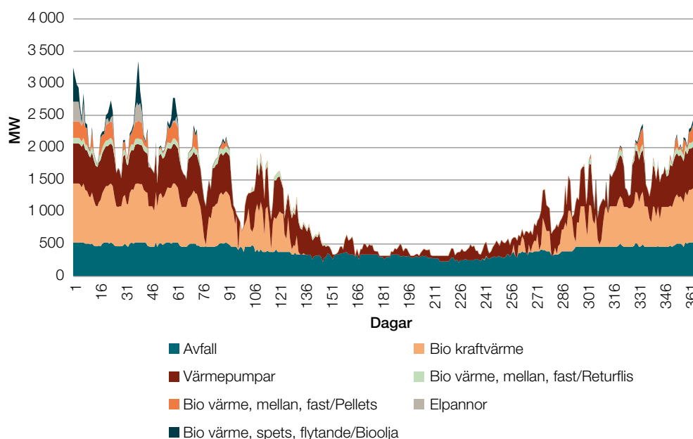
Figur 41. Fjärrvärmeproduktion i Stockholmsområdet.
