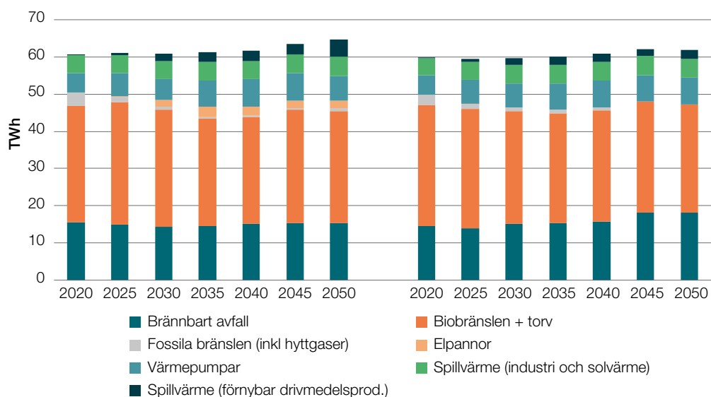
Figur 8. Fjärrvärmeproduktion per energislag i basfall (vänster) jämfört med utfasning av kraftvärme (höger).
