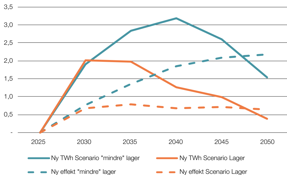
Figur 6. Utbyggnad av ny kraftvärme (effekt) samt ny produktion (TWh) beroende på antaganden om lager och livstidsförlängning av kärnkraft, jämfört med 2025.
