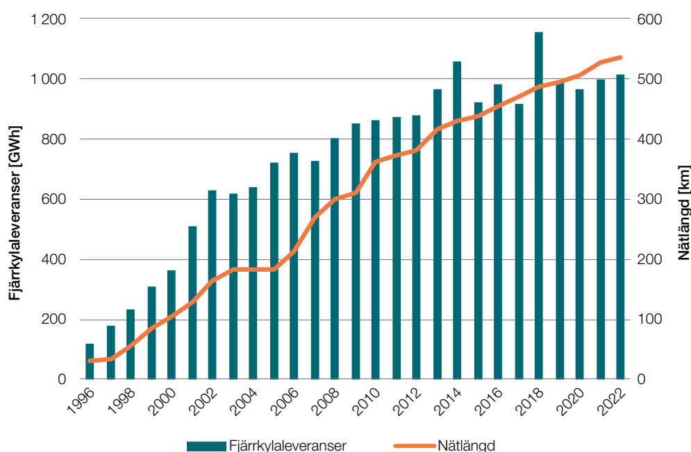
Figur 44. Svenska fjärrkylaleveranser och nätutbyggnad, 1996–2022.
