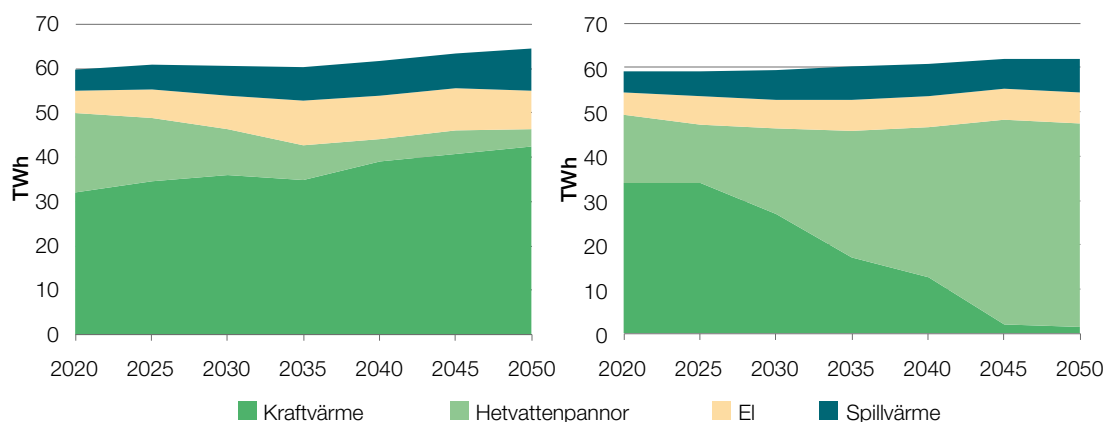
Figur 9. Fjärrvärmeproduktionsmixens olika delar, basfall (vänster), utfasning av kraftvärme (höger).
