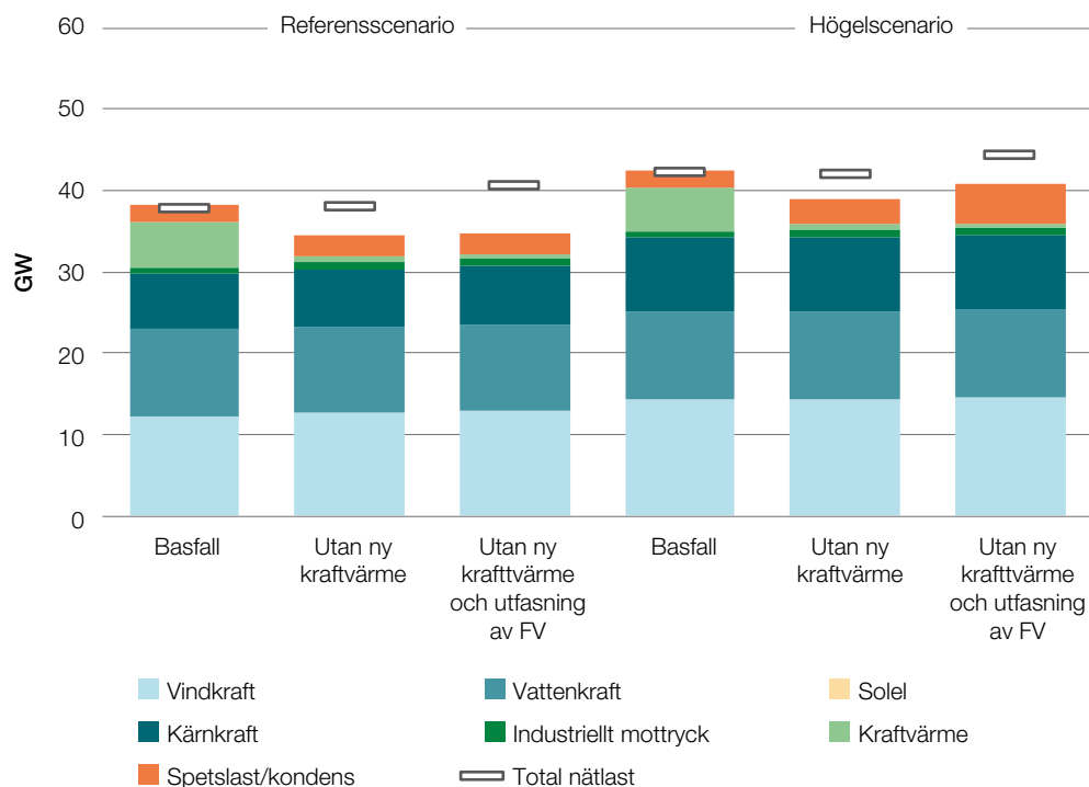
Figur 10. Eleffektbalansen under vinterdagseftermiddagen olika beräkningsfall (modellår 2040).
