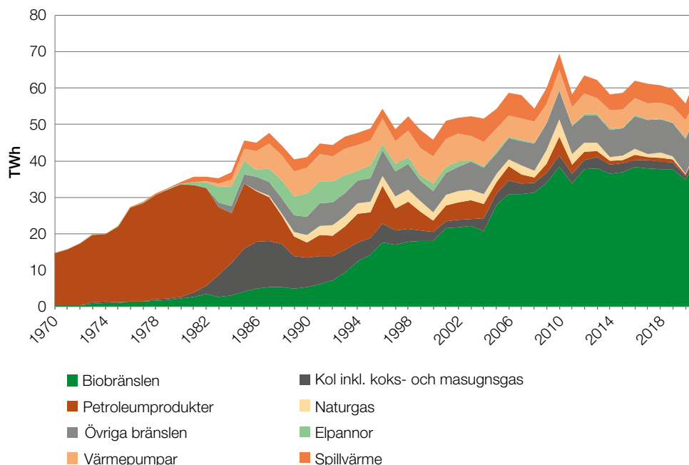
Figur 40. Tillförd energi för fjärrvärmeproduktion från 1970, TWh.
