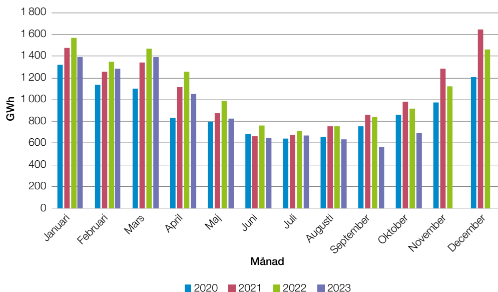
Figur 27. Månadsvis förnybar kraftvärmeproduktion, GWh.
