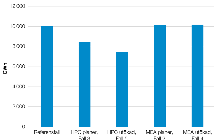
Figur 37. Årlig elproduktion från kraftvärme (i fjärrvärmenäten), för år 2035.
