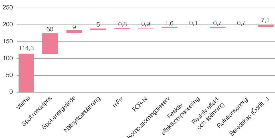
Figur 19. Påverkan på typlanläggningens lönsamhet från att bidra med olika förmågor. Ersättningarna i figuren utgörs av en mix av intäkter från befintliga marknader (energivärde, nätnytttoersättning, mFRR, FCR-N, kompletterande störningsreserv) och alternativkostnad, Öre/kWh.
