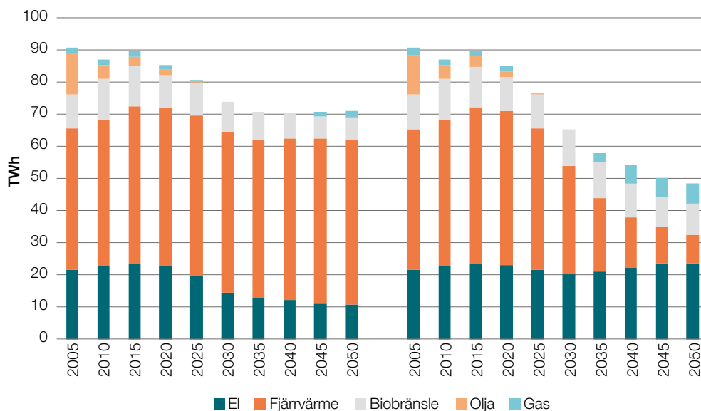
Figur 3. Slutlig energianvändning för uppvärmning (inklusive varmvattenberedning) inom bostäder och service. Basfallet till vänster och fjärrvärmeutfasningsfallet till höger.
