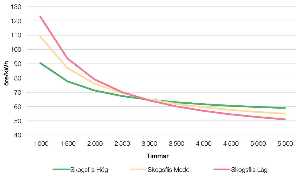
Figur 13. Genomsnittlig produktionskostnad vid olika antal fullasttimmar för ett biokraftvärmeverk som använder skogsflis som bränsle. Anläggningsstorlekarna är 10, 25 respektive 40 MW i scenarierna Låg, Medel och Hög.
