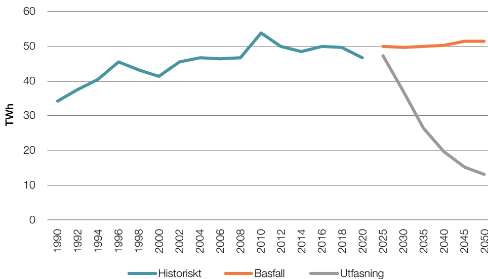
Figur 2. Utfasningen av fjärrvärme (grå linje) jämfört med basfallet (orange linje), TWh.
