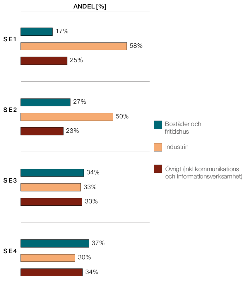
Figur 7 Elanvändning uppdelat på sektorer och elområde avseende år 2022, procent Källa: SCB Elanvändning i Sverige efter användningsområde (SNI 2007) och elområde. År 2015 - 2022. PxWeb (scb.se)
