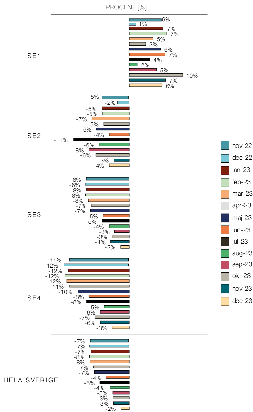
Figur 9 Förändring av temperatur- och kalenderkorrigerad elanvändning jämfört med motsvarande elanvändningen under referensperioden (senaste 5 åren)
