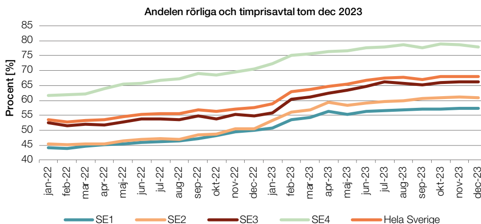
Figur 17 Utveckling av andel rörliga elhandelsavtal och timprisavtal t.o.m. november 2023
