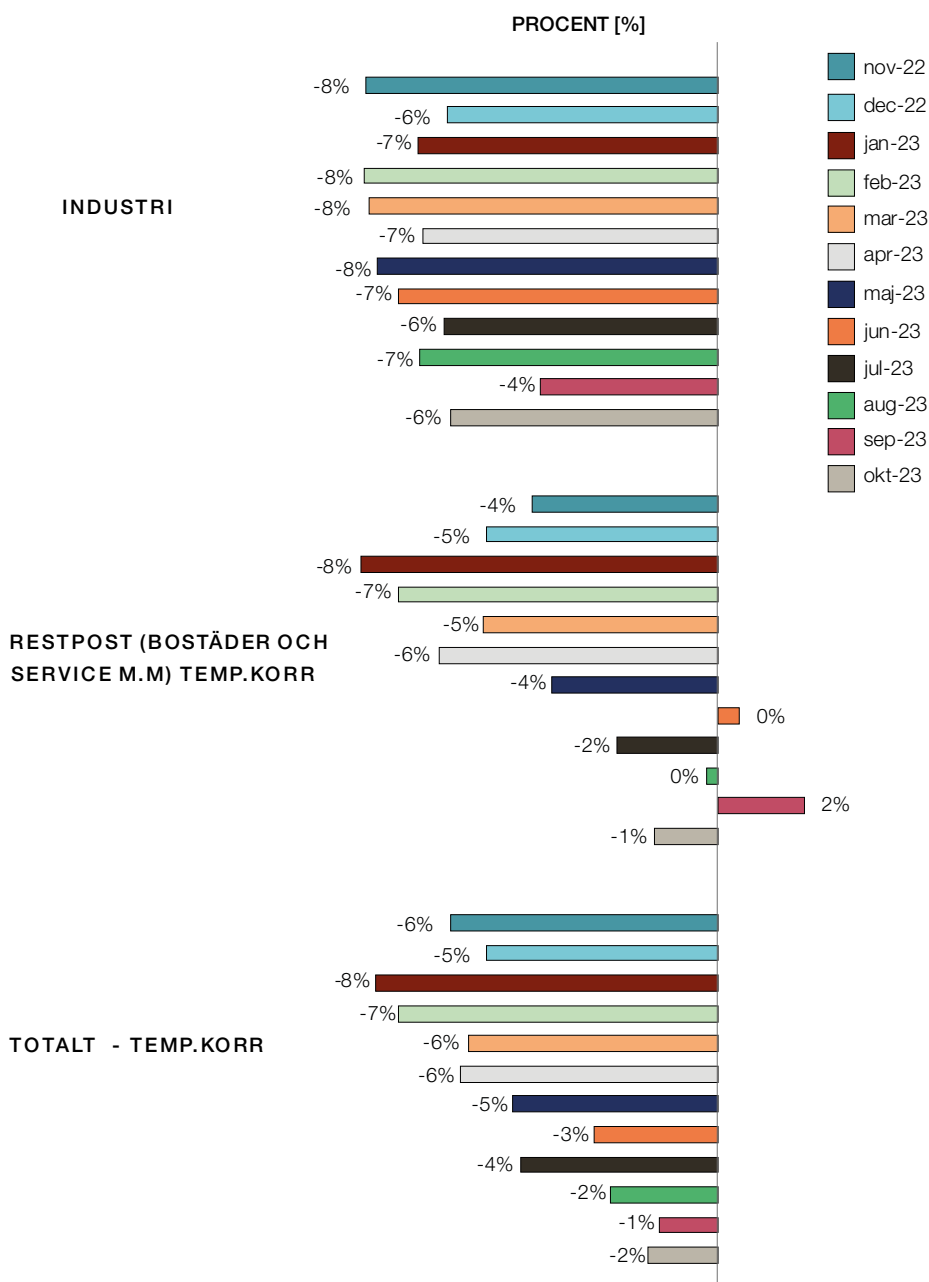
Figur 11 Förändring av den faktiska elanvändningen uppdelat per sektor jämfört med referensperioden (senaste 5 åren).
