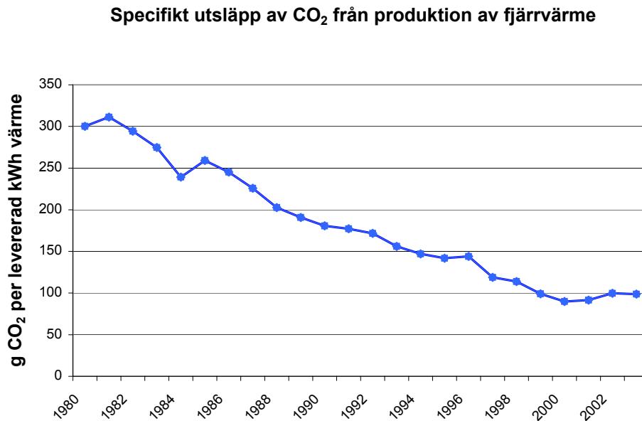
Figur 4 Specifika utsläpp av koldioxid från produktion av fjärrvärme
