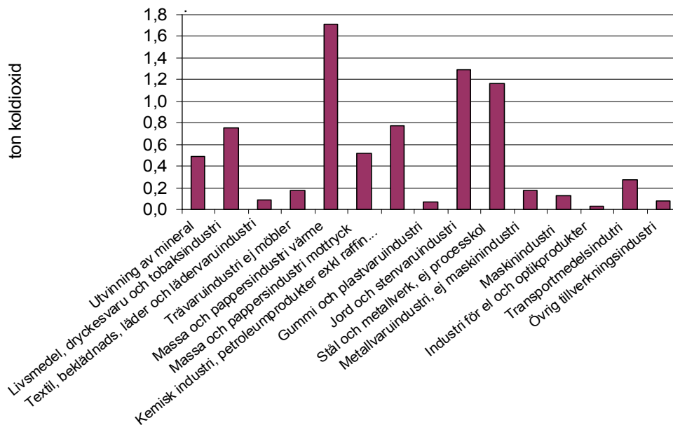
Figur 17 Koldioxidutsläpp i industrin fördelat på branscher
