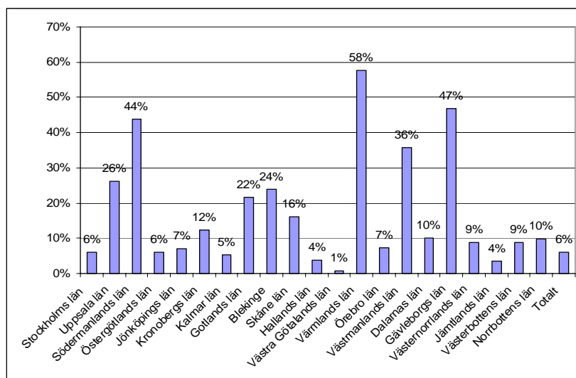
Figur 38 OFFROTEN: Den totala minskningen av den årliga energiförbrukningen för hela landet ligger på 6 procent men varierar stort mellan länen
