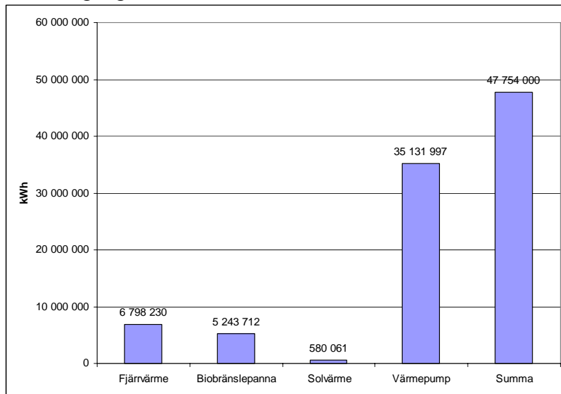
Figur 29 OFFROT Beräknad årlig energibesparning för olika konverteringslag
