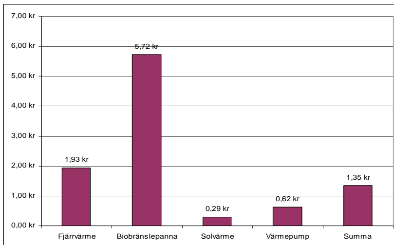
Figur 39 OFFROTEN: Annualiserade investeringskostnaderna per besparad kWh per år över livstiden, där livstiden antas vara 20 år för fjärrvärme, 25 år för solvärme samt 15 år för biobränslepanna och värmepump. Räntan ligger på 4,8 procent, inga underhållskostnader
