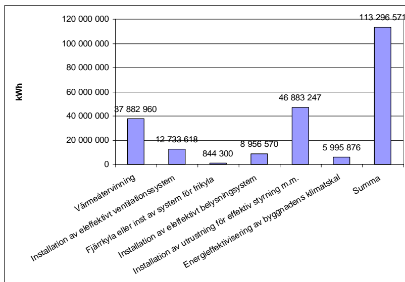
Figur 30 OFFROT: Beräknad årlig energibesparning för andra åtgärder än byte av uppvärmningssystem
