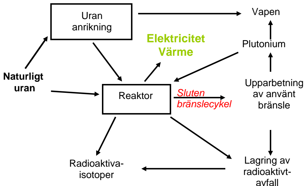
Figur 1 Generaliserad kärnbränslecykel. Vid en öppen cykel går radioaktivt avfall från reaktorn direkt till lagring. Vid en slutna cykel upparbetas och återanvänds använt bränsle.
