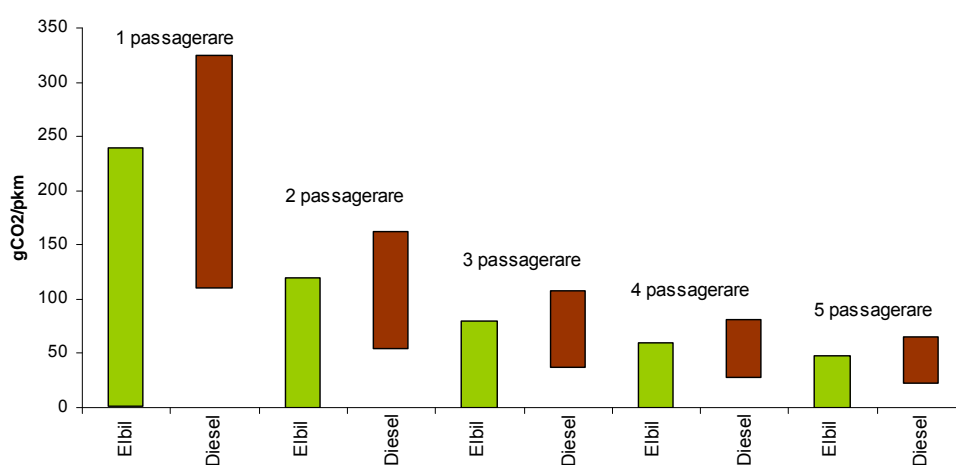
Figur 3 - Koldioxidutsläpp som funktion av fordonsbeläggning. Jämförelse av en elbil och en mycket energieffektiv dieselbil ur olika perspektiv på beräkning av utsläppen.
