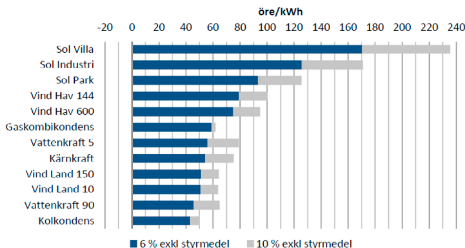
Figur II. Elproduktionskostnader för kommersiella tekniker som enbart producerar el, exkl. styrmedel med 6 respektive 10 % kalkylränta
