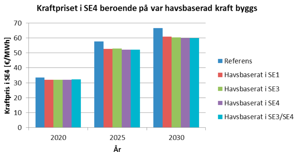
Figur 31 Elpriset i SE4 beroende på var den havsbaserade vindkraften byggs. Alla resultat är från modellerade scenarier med högt bränslepris.
