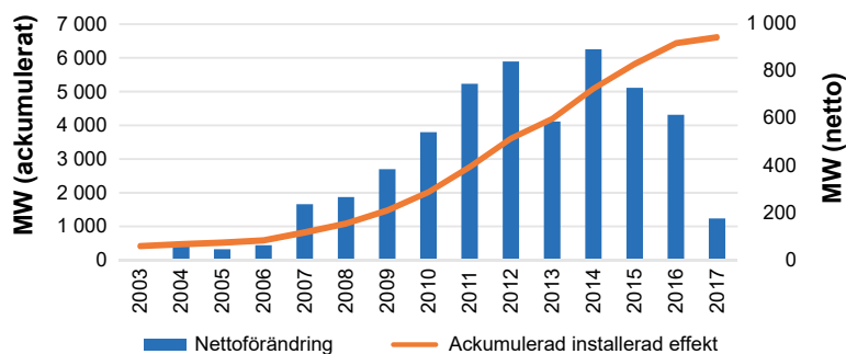
Figur 2. Årlig ackumulerad och årlig nettoförändring av installerad effekt vindkraft, MW.
