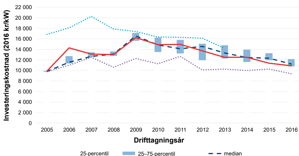
Figur 13. Investeringskostnader för vindkraftsprojekt som tagits i drift perioden 2005–2016, 2016 kr/kW.
