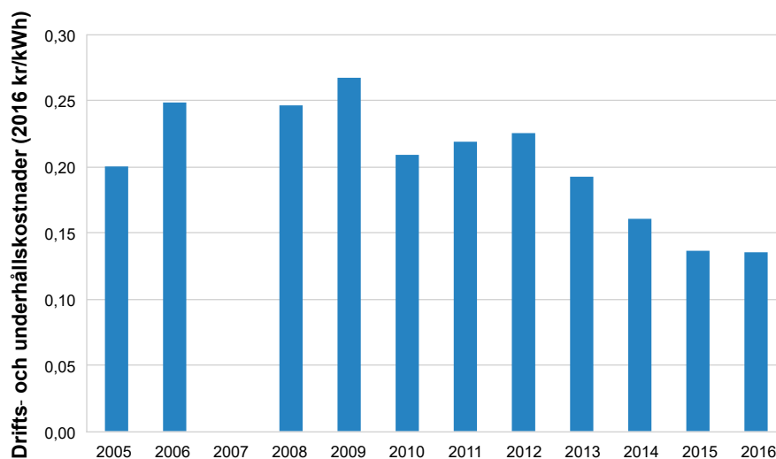
Figur 15. Drifts- och underhållskostnadernas utveckling under perioden 2005–2016, 2016 kr/kWh.
