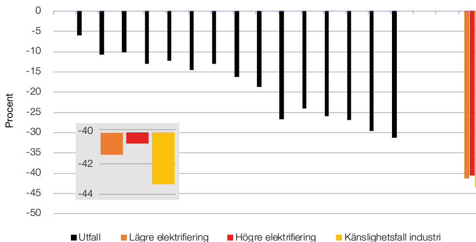
Figur 36. Förändrad energiintensitet i förhållande till basåret (2005), för åren 2005–2020 samt år 2030 i scenarier och känslighetsfall, procent.
