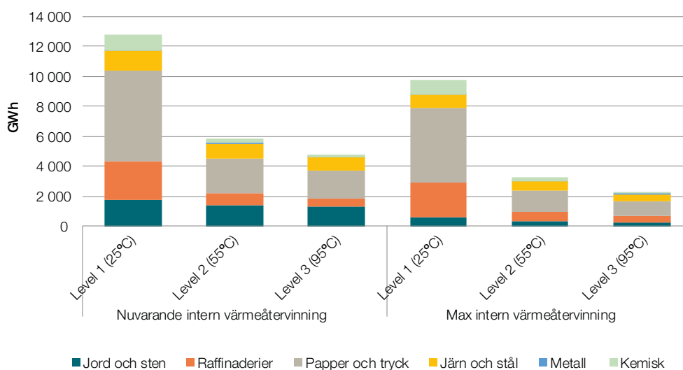
Figur 43. Industriell spillvärmepotential i Sverige för olika temperaturnivåer och grad av intern värmeåtervinning enligt projektet Seenergies (baserat på 2015).
