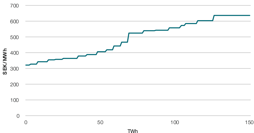
Figur 38. Produktionskostnad för ny vindkraft i Sverige, givet 25 års livslängd och 6 procent kalkylränta (real).
