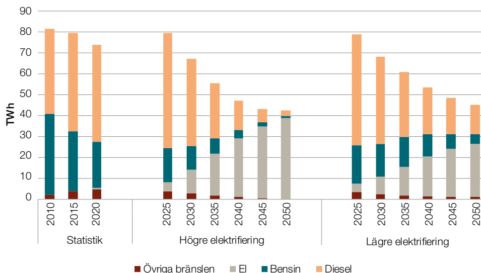
Figur 13. Energianvändning 2010–2020 samt 2020–2050 inom vägtrafiken uppdelad på olika bränslen vid scenarierna Högre elektrifiering och Lägre elektrifiering , TWh.
