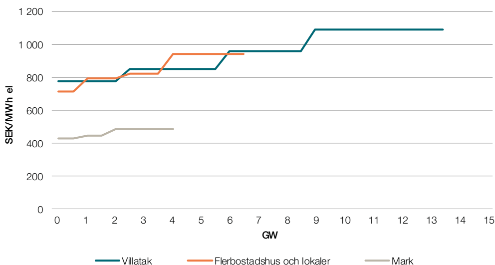
Figur 39. Produktionskostnader och potential för solcell i Sverige på villatak, flerbostadshus och lokaler och på mark.
