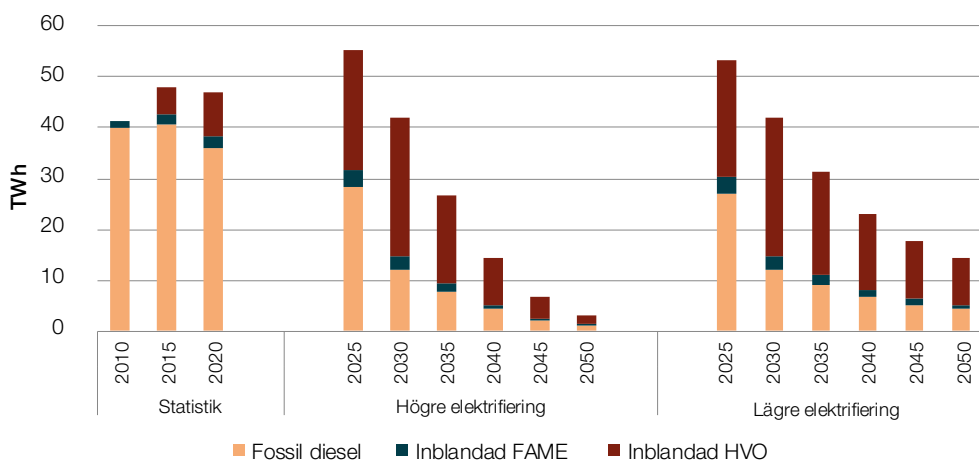
Figur 15. Energianvändning inom transportsektorn i scenarierna Högre elektrifiering och Lägre elektrifiering för diesel och låginblandade biodrivmedel 2010–2020 samt 2020–2050, TWh.
