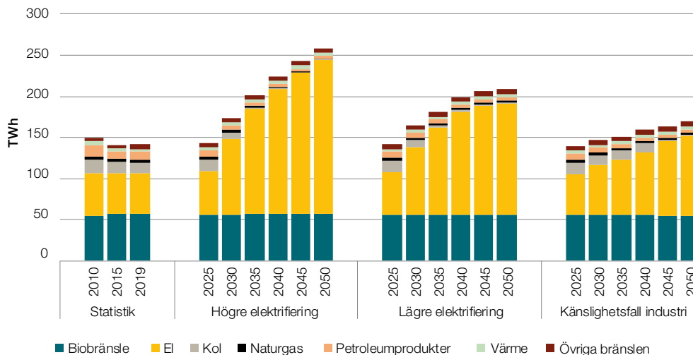
Figur 6. Industrins energianvändning per energibärare 2010, 2015, 2019 samt 2025–2050 för scenarierna Högre elektrifiering , Lägre elektrifiering och Känslighetsfall industri , TWh.
