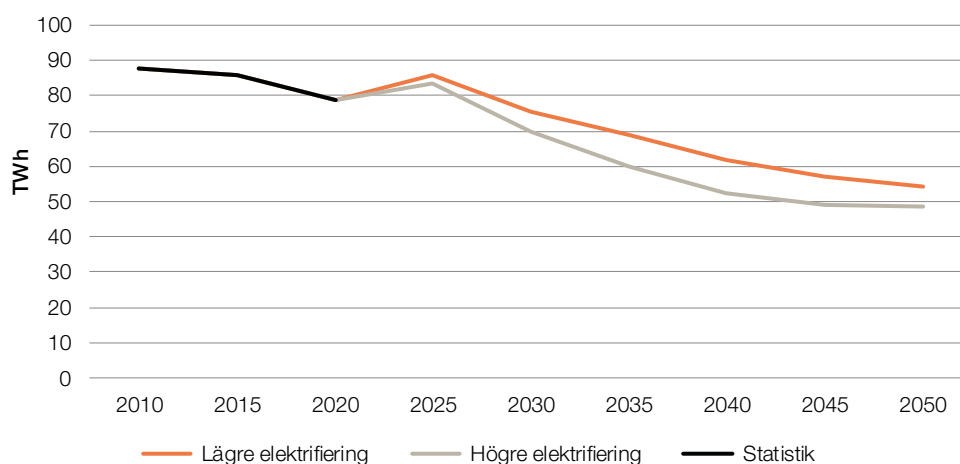
Figur 12. Total energianvändning, inrikes transporter, 2010–2020 samt 2020–2050 för de olika scenarierna, TWh.
