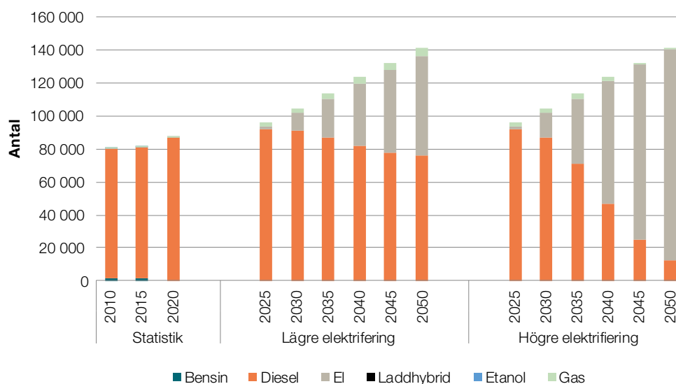
Figur 17. Antal tunga lastbilar i fordonsflottan uppdelat på drivlina 2010–2020 samt 2020–2050 vid scenarierna Lägre elektrifiering och Högre elektrifiering .
