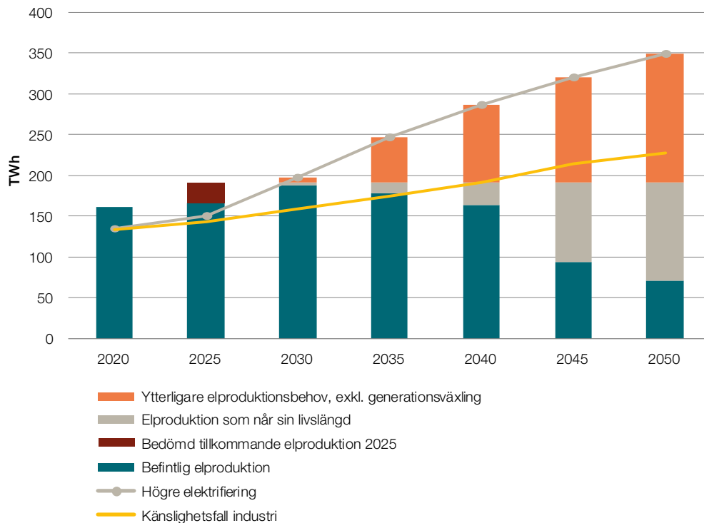
Figur 27. Ökning av elbehovet till 2050 (utfallsrummet visar skillnaden mellan Högre elektrifiering och Känslighetsfall industri ) i jämförelse med befintlig elproduktion, antagande om elproduktion 2025 och ytterligare behov för att nå det högre utfallet.
