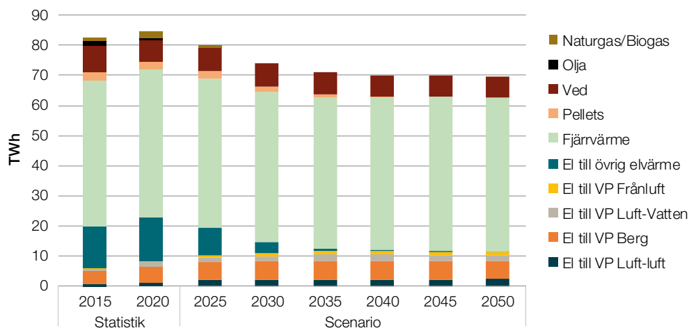
Figur 20. Köpt energi till bostäder och lokalers uppvärmning och varmvatten, historisk utveckling 2015–2020 och förväntad energiåtgång 2025–2050 uppdelat på energislag, TWh.
