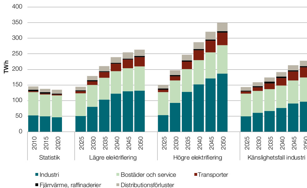
Figur 26. Elanvändning uppdelat per sektor 2010, 2015 och 2020 samt per scenario 2025–2050, TWh.
