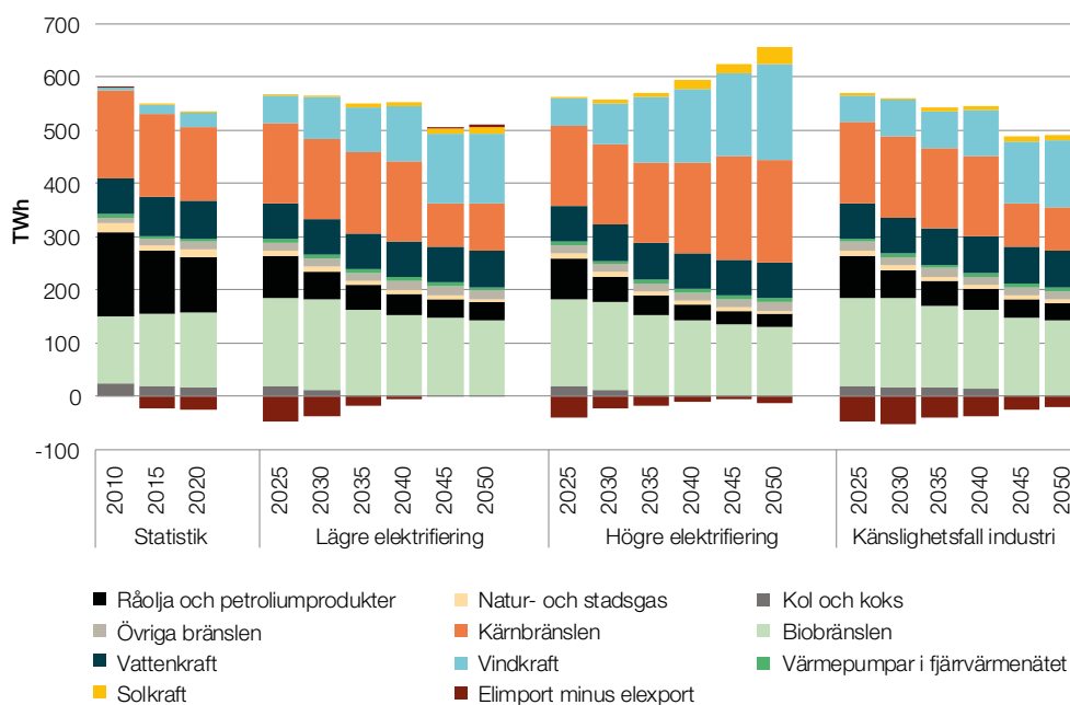
Figur 3. Energitillförsel (inkl. nettoimport/export) per energibärare 2010, 2015 och 2020 samt i scenarierna till 2050, TWh.
