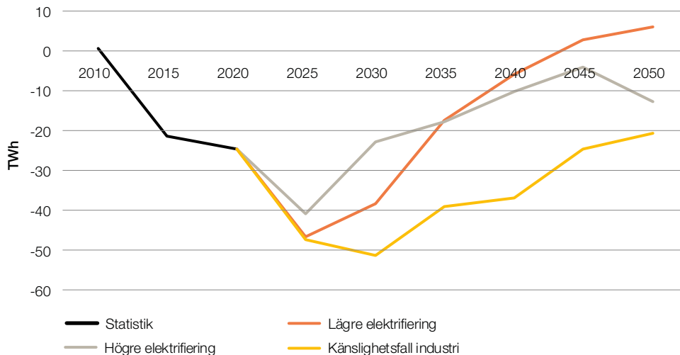
Figur 30. Nettohandel för Sverige i de olika scenarierna, nettoexport (-) och nettoimport (+), TWh.
