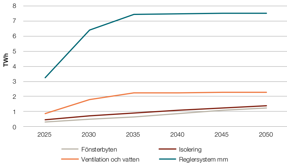
Figur 21. Olika energieffektiviseringsåtgärders förväntade bidrag till minskat nettoenergibehov 2025–2050, TWh.
