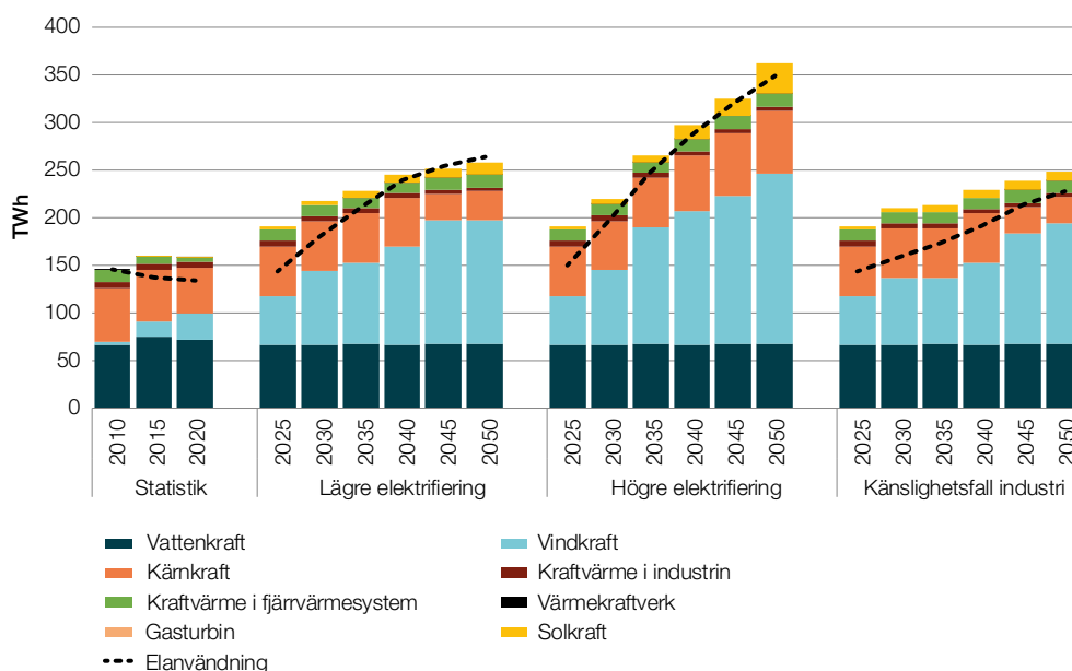
Figur 28. Elproduktion uppdelat på produktionslag och elanvändning 2010, 2015, 2020 samt i de olika scenarierna 2025–2050, TWh.
