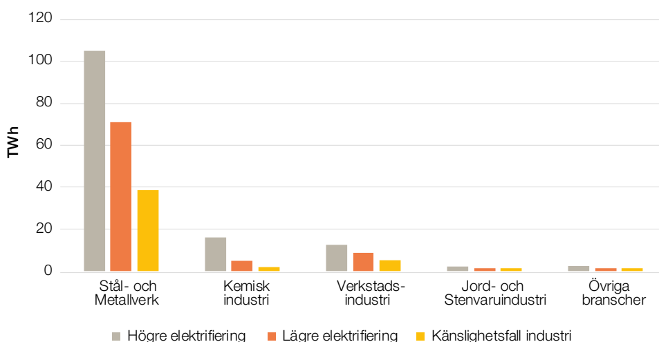
Figur 10. Tillkommande el i TWh för olika branscher 2050 jämfört med 2019.
