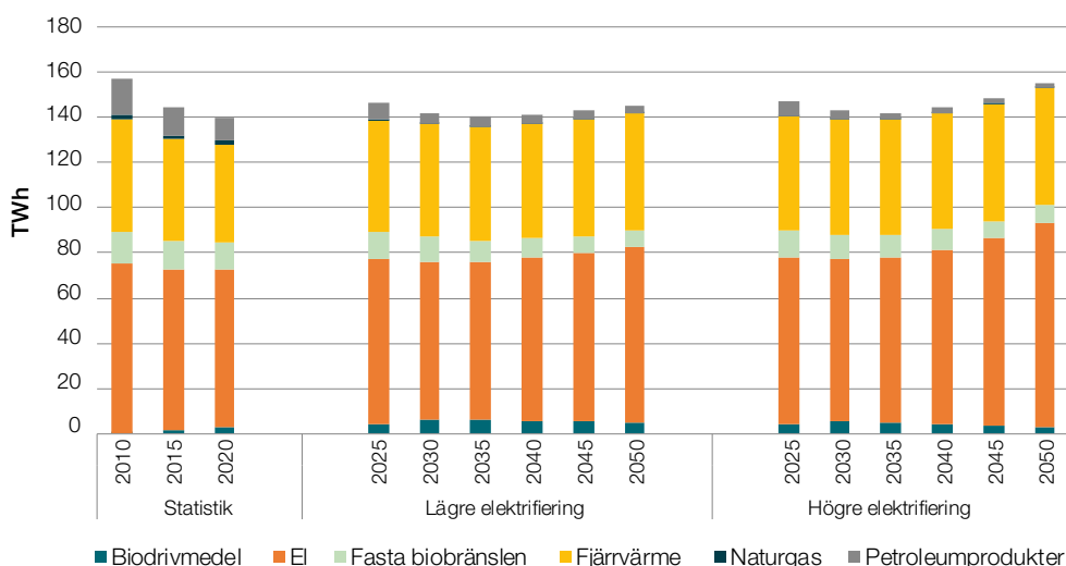
Figur 18. Total slutlig energianvändning 2010–2020 samt 2020–2050 i scenarierna Lägre elektrifiering och Högre elektrifiering uppdelat på energislag, TWh.
