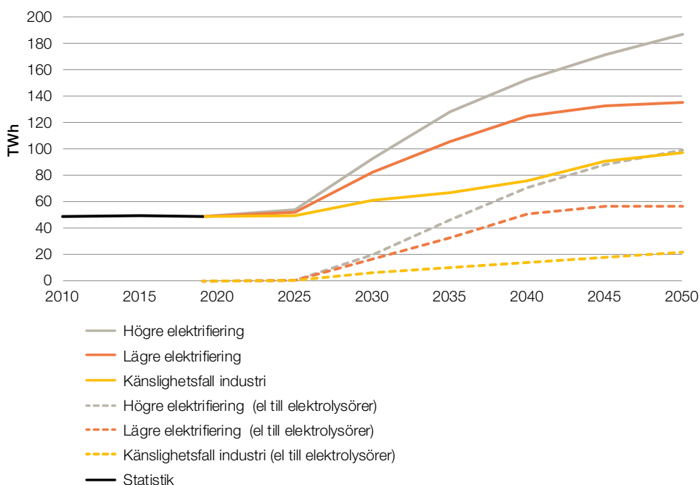
Figur 7. Industrins elanvändning 2010–2019 och scenariernas utfallsrum för elanvändningen samt el till elektrolysörer 2020–2050, TWh.
