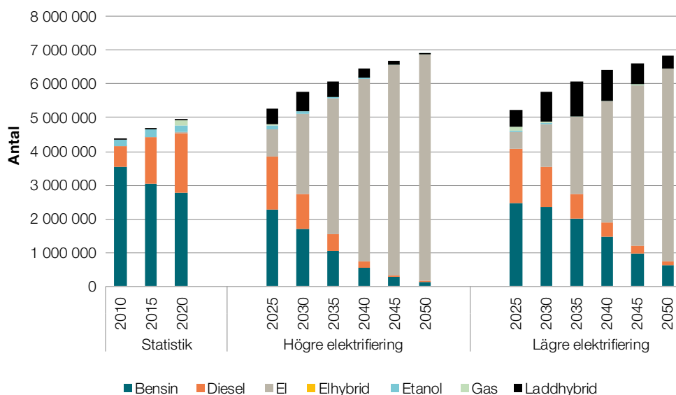
Figur 16. Antal personbilar i fordonsflottan uppdelat på drivlina 2010–2020 samt 2020–2050 vid scenarierna Högre elektrifiering och Lägre elektrifiering .
