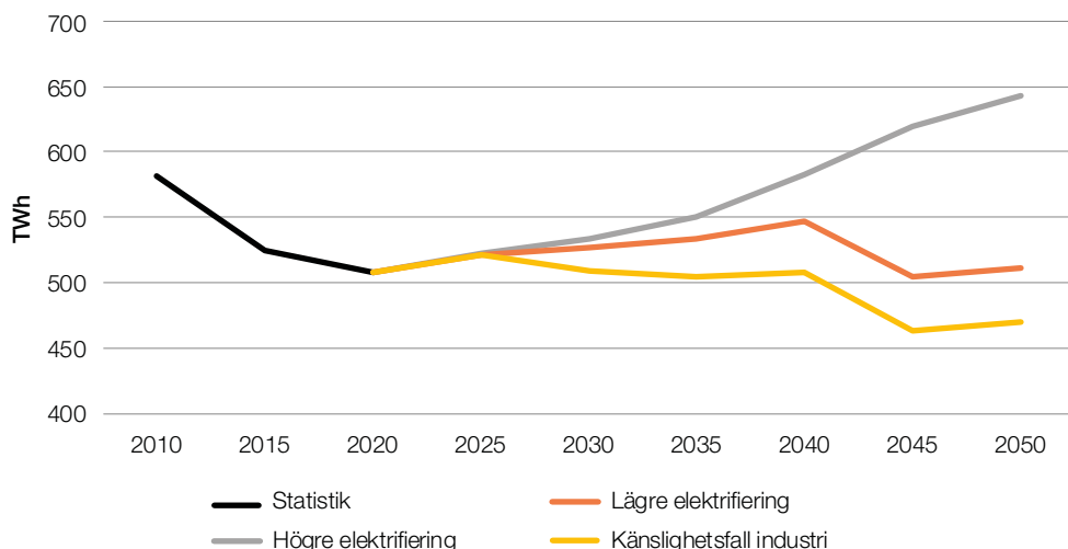
Figur 1. Total energitillförsel (inkl. nettoimport/export) 2010, 2015 och 2020 samt i scenarierna till 2050, TWh.
