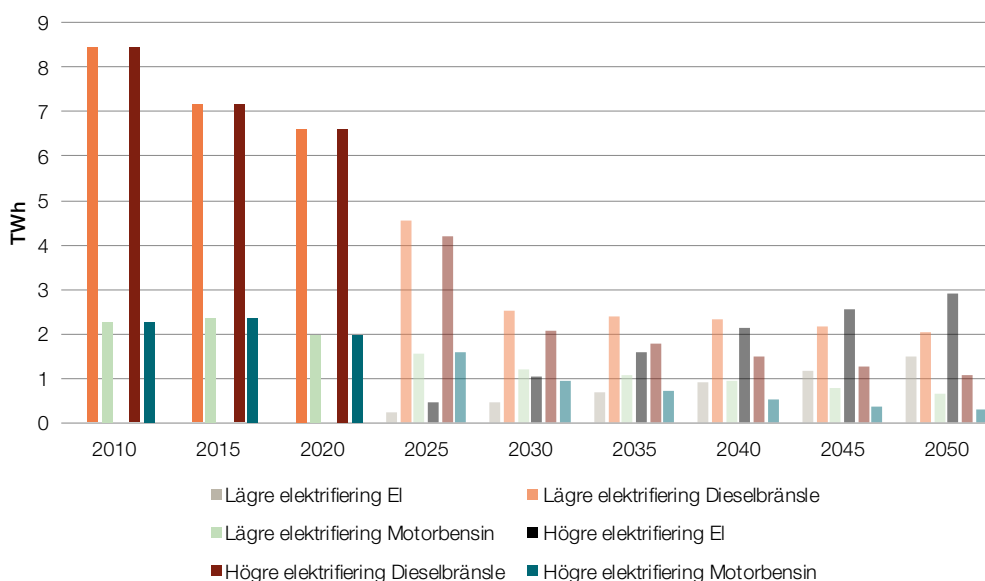
Figur 23. Utvecklingen av användning av diesel, motorbensin och el till arbetsmaskiner 2010–2020 samt i de olika scenarierna 2025–2050, TWh.
