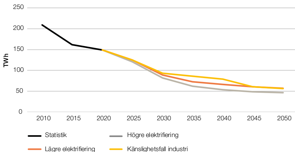
Figur 2. Tillförsel av fossila bränslen 2010, 2015 och 2020 samt i scenarierna till 2050, TWh.
