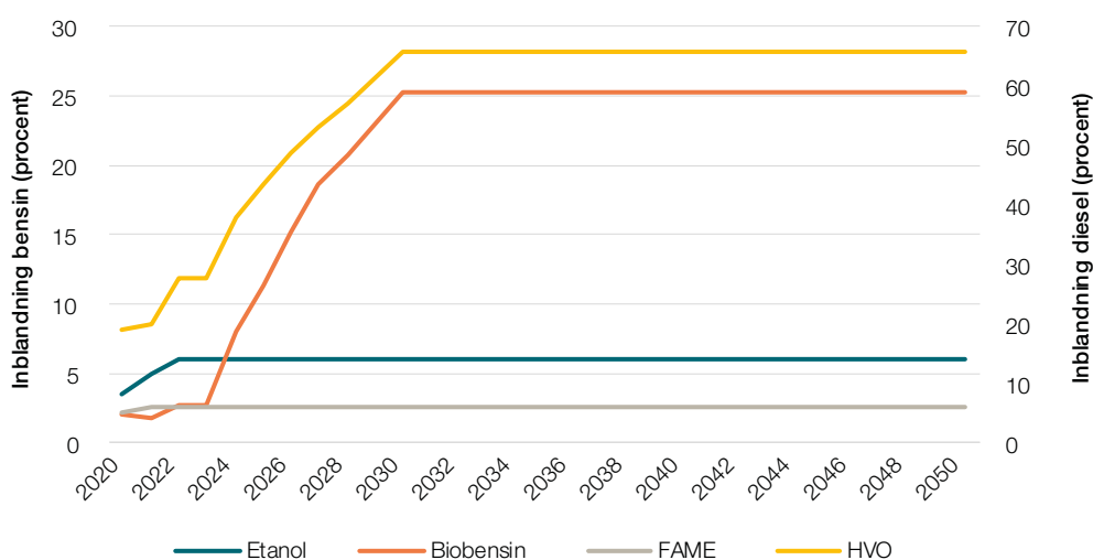
Figur 44. Inblandningsnivåer i bensin och diesel, 2020–2050, energiprocent.
