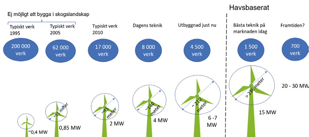
Figur 29. Räkneexempel över hur många vindkraftverk som krävs för att producera 100 TWh med olika turbintekniker.
