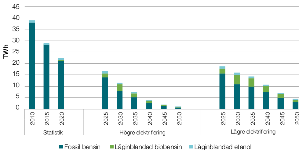
Figur 14. Energianvändning inom transportsektorn i scenarierna Högre elektrifiering och Lägre elektrifiering för bensin och låginblandade biodrivmedel 2010–2020 samt 2020–2050, TWh.
