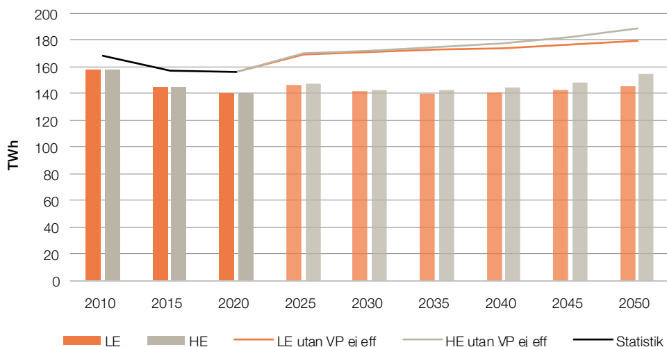
Figur 22. Jämförelse och illustration av hur det skulle se ut utan värmepumpar och om inga energieffektiviseringsåtgärder genomförs från 2020, TWh.
