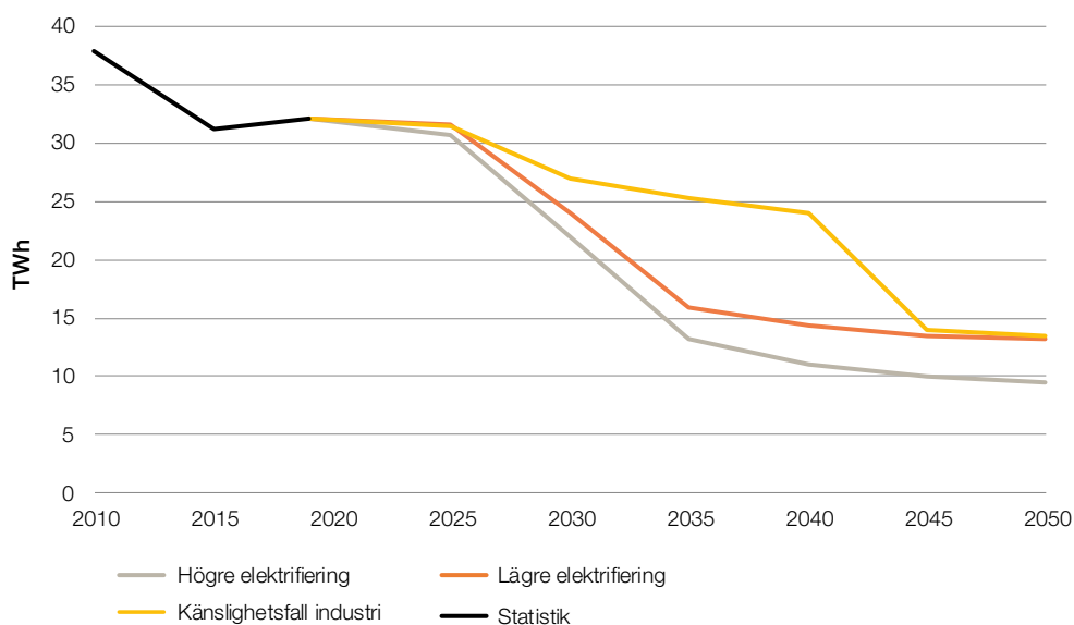
Figur 8. Industrins användning av fossila bränslen 2010–2019 och utfallsrum 2020–2050, TWh.
