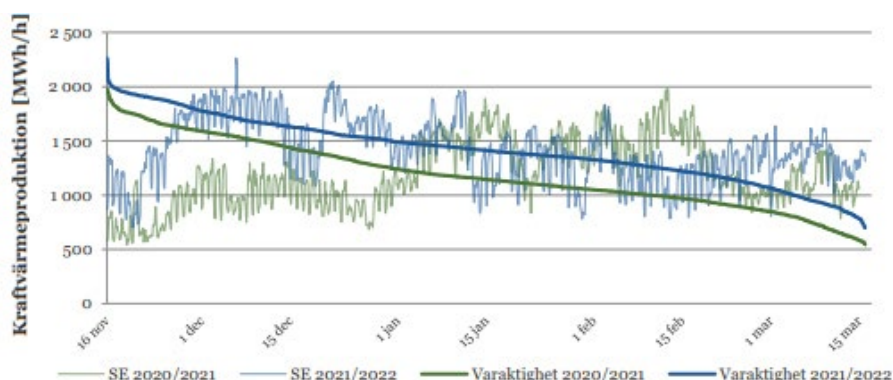
Figur 1. Timmedelvärden för den svenska kraftvärmeproduktionen under de vintrarna 2020/2021 och 2021/2022 vintrarna
