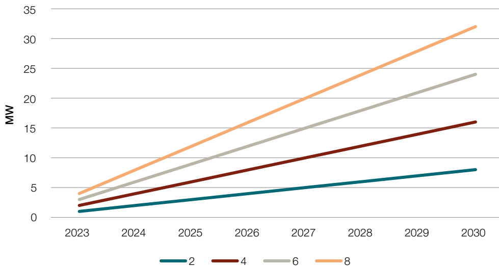
Figur 10. Total installerad effekt givet ORC-turbin på 500 kW och antal installationer per år (2, 4, 6 eller 8)
