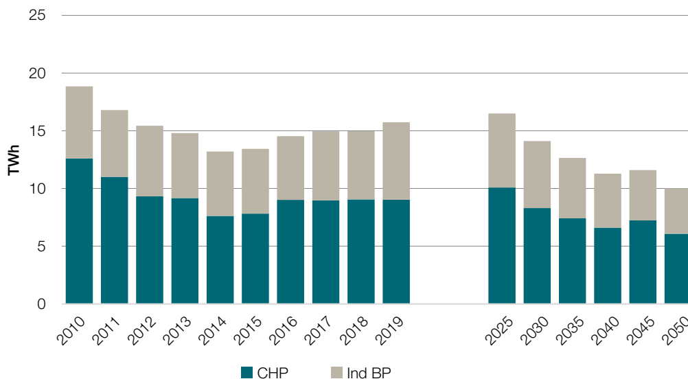
Figur 58. Utvecklingen av kraftvärmeproducerad el i scenario FF55
