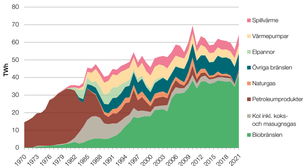
Figur 16. Tillförd energi för fjärrvärmeproduktion fr.o.m. 1970, TWh
