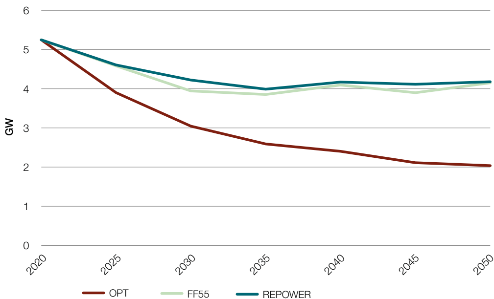
Figur 56. Medeleffektbehov för individuell eluppvärmning – vinterdag
