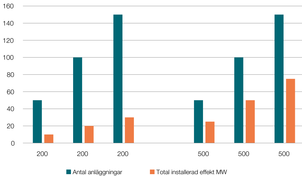
Figur 9. Total effekt beroende på antagande om installering av ORC turbiner på 200 MW och 500 MW effekt, beroende på hur många företag som installerar.
