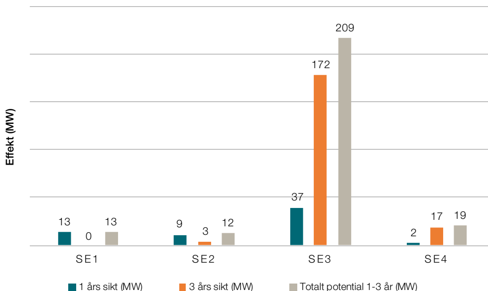
Figur 6. Elproduktionspotential kalla vinterdagar i befintlig kraftvärme 1 resp. 3 års sikt
