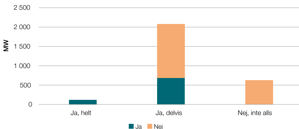
Figur 8. Tekniska möjligheter till kylförmåga, svarande i Svebios biokraftundersökning 2022, (av svarande med effekt på 2 800 MW)
