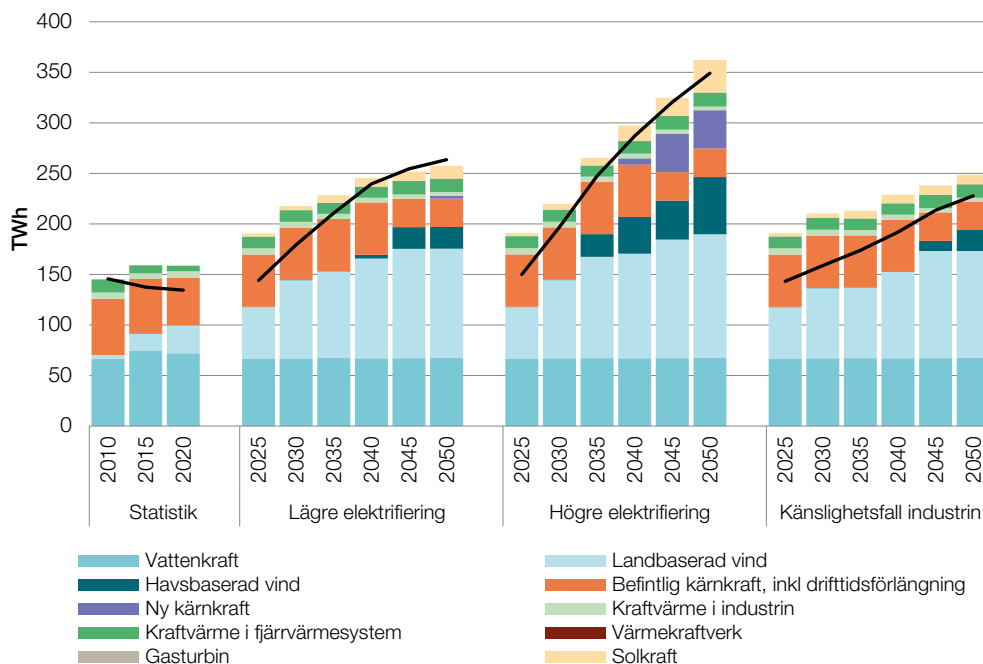
Figur 21. Elproduktion uppdelat på produktionsslag och elanvändning i de olika scenarierna 2025–2050, TWh.
