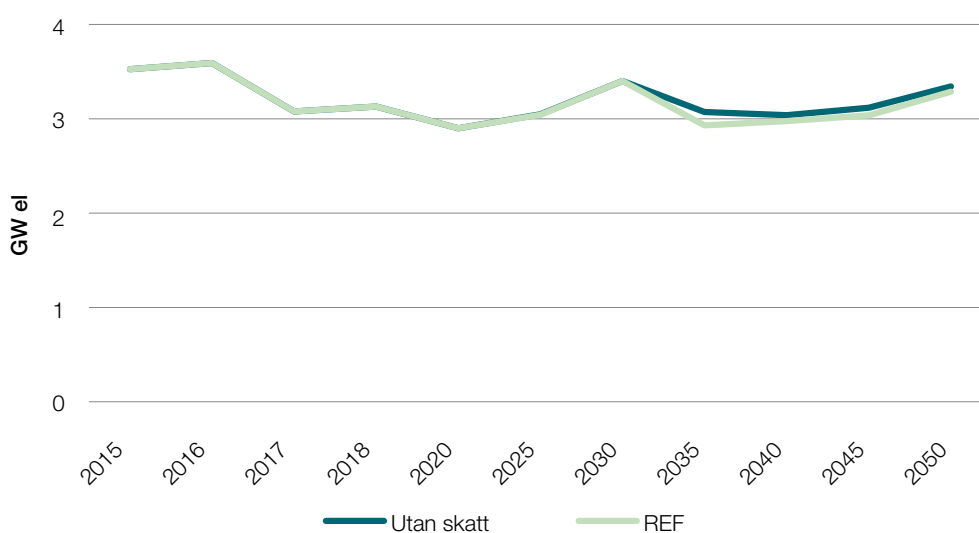
Figur 44. Installerad kraftvärmekapacitet i de två beräkningsfallen samt statistik mellan 2015–2020
