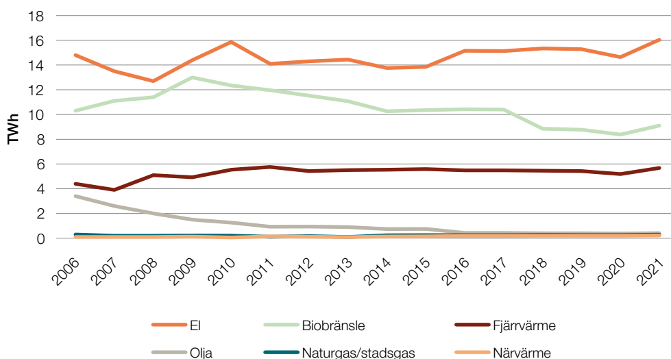
Figur 13. Total energianvändning för uppvärmning och varmvatten i småhus fördelad på energikällor och energibärare, år 2006–2021, TWh.
