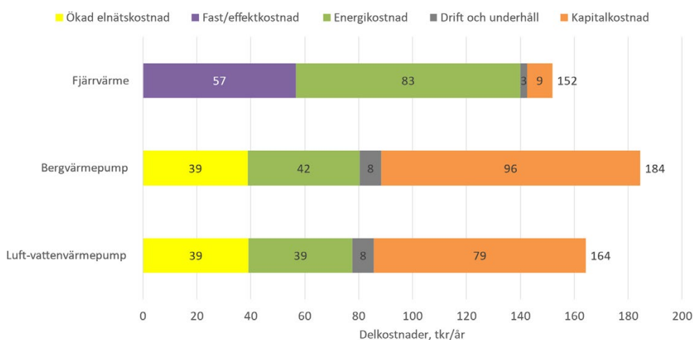
Figur 33. Årliga kostnader för uppvärmning 2022 för elprisområde SE3 för fjärrvärme, bergvärme samt luft-vattenvärmepump, uttryckt i tusentals kronor per år utan moms.
