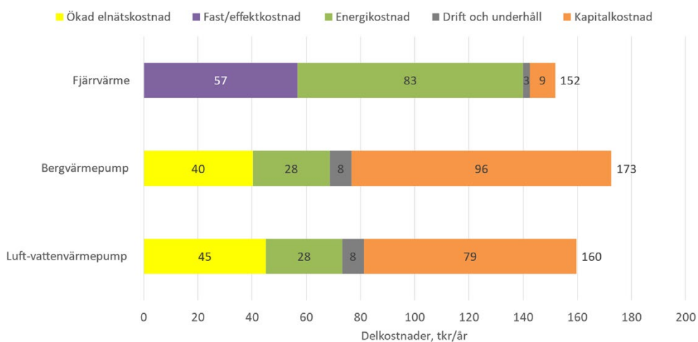
Figur 32. Årliga kostnader för uppvärmning 2022 för elprisområde SE2 för fjärrvärme, bergvärme samt luft-vattenvärmepump, uttryckt i tusentals kronor per år utan moms.
