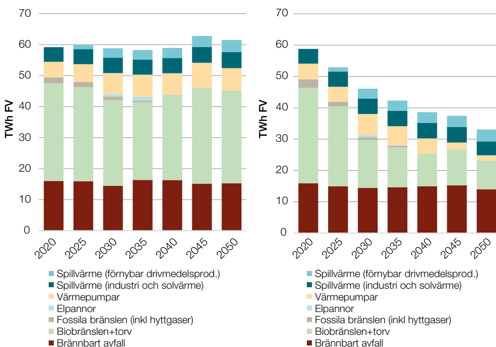
Figur 55. Fjärrvärmeproduktion scenario OPT (vänster) jämfört med Scenario FF55 (höger)
