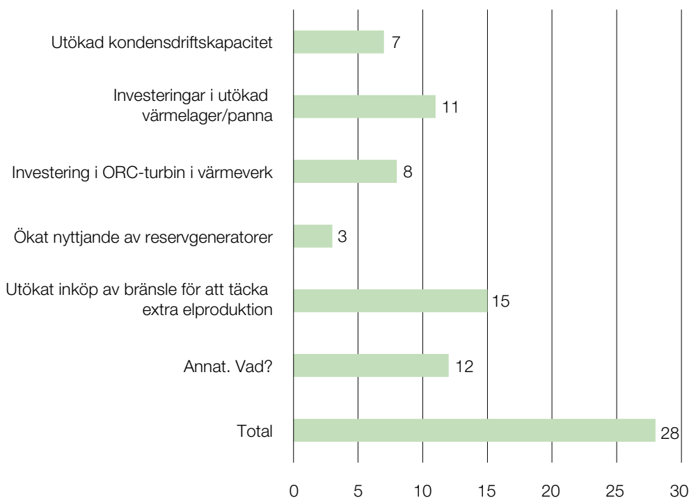
Figur 7. Tekniska åtgärdsbehov för att möjliggöra ökad produktion av el från kraftvärme kalla vinterdagar vid hög efterfrågan på el
