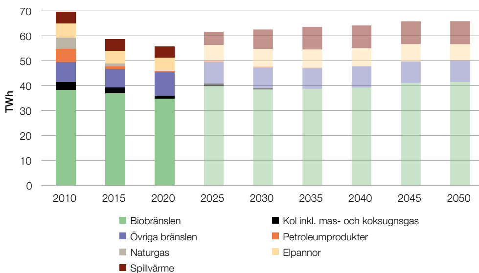
Figur 23. Tillförd energi för fjärrvärmeproduktion för scenario Lägre elektrifiering till 2050, TWh.
