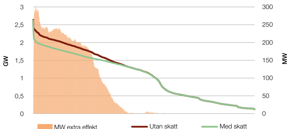
Figur 43. MW extra effekt (Sekundäraxel) vid fallet med borttagen koldioxidskatt för 2020 års energipriser och obegränsade backningsmöjligheter
