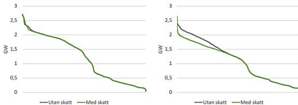
Figur 42. Varaktigheten för elproduktion i kraftvärmeverken under helåret 2022 i ett fall där backningsmöjligheterna antas vara begränsade i kombination med 2022 års bränslepriser (till vänster) och ett fall där backningsmöjligheterna antas vara obegränsade i kombination med 2020 års bränslepriser (till höger)
