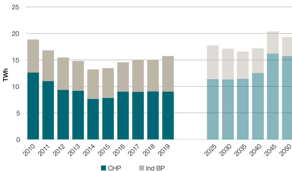
Figur 57. Utvecklingen av kraftvärmeproducerad el i referensfallet (scenario OPT)
