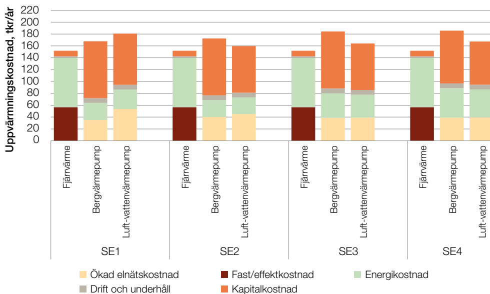
Figur 39. Konkurrensjämförelse mellan fjärrvärme, bergvärme och luft-vattenvärmepump för en villa 2022, uppdelat på olika elprisområden.
