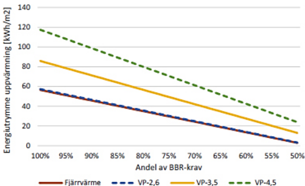
Figur 46. Kvarvarande energitrymme för uppvärmning i ett flerbostadshus varmt med fjärrvärme och tre olika hus värmda med värmepumpar med olika prestanda (SCOP på 2,6, 3,5 och 4,5).
