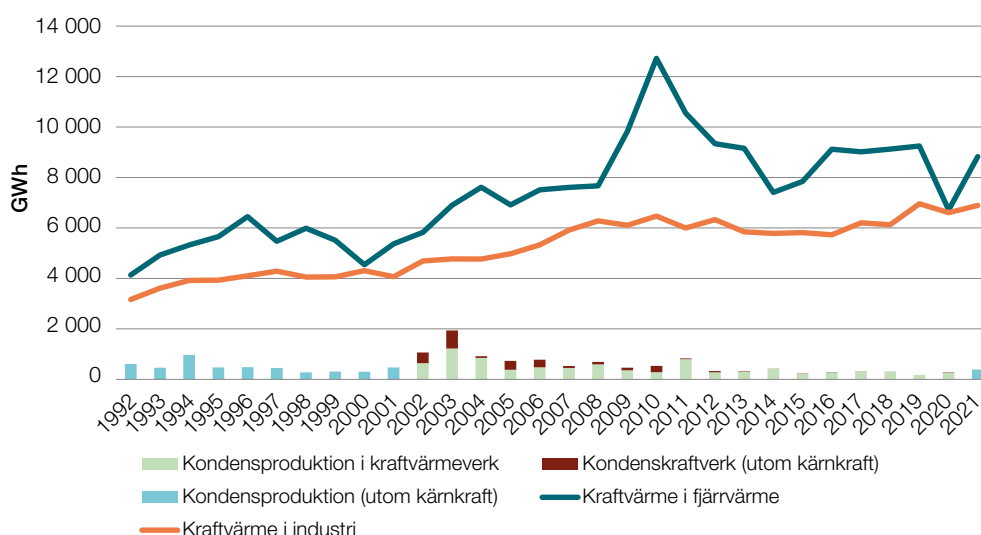
Figur 17. Kraftvärmeproducerad el och kondenskraft, GWh.
