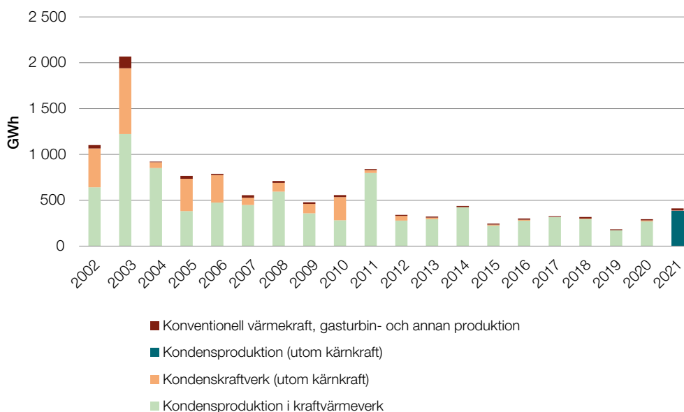
Figur 18. Kondensproduktion (ej kärnkraft), inkl. gasturbiner, GWh.
