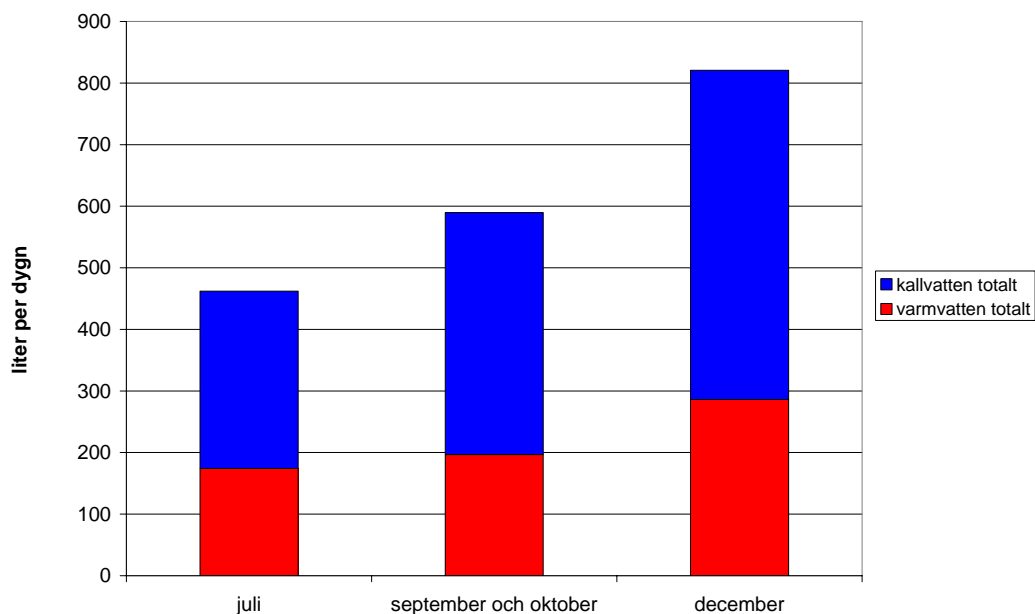
Bilaga G.2 Genomsnittlig total varm- och kallvattenanvändning per dygn (inklusive wc och övrig vattenanvändning) olika mät månader i hushåll J (barnfamilj i villa)
