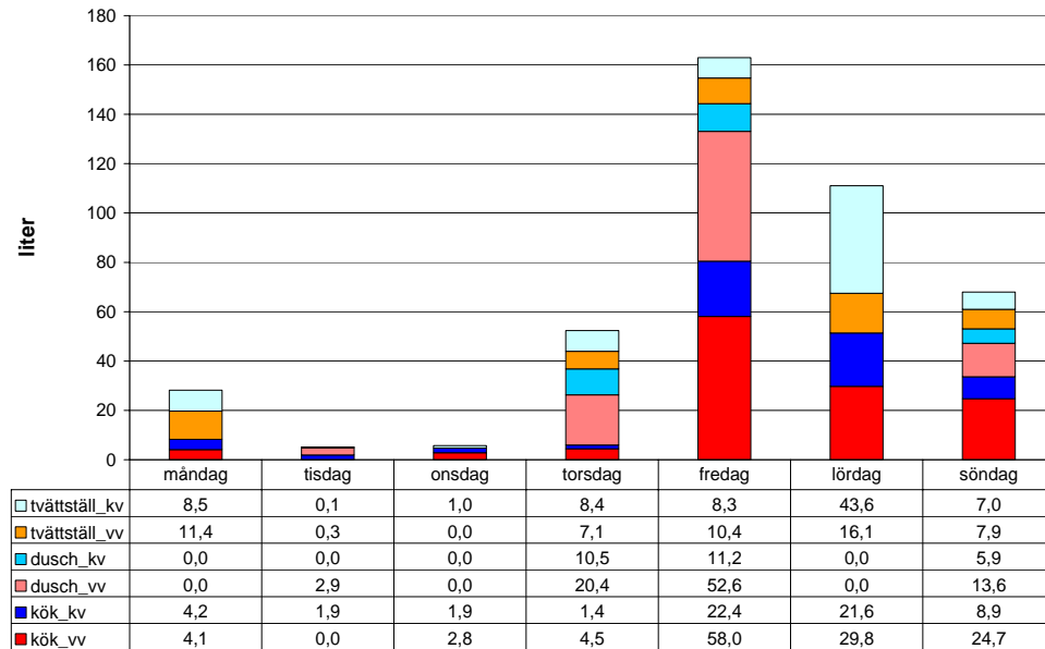
Figur 5.5 Användning av varm- och kallvatten under en vecka i hushåll A (singel i lägenhet)
