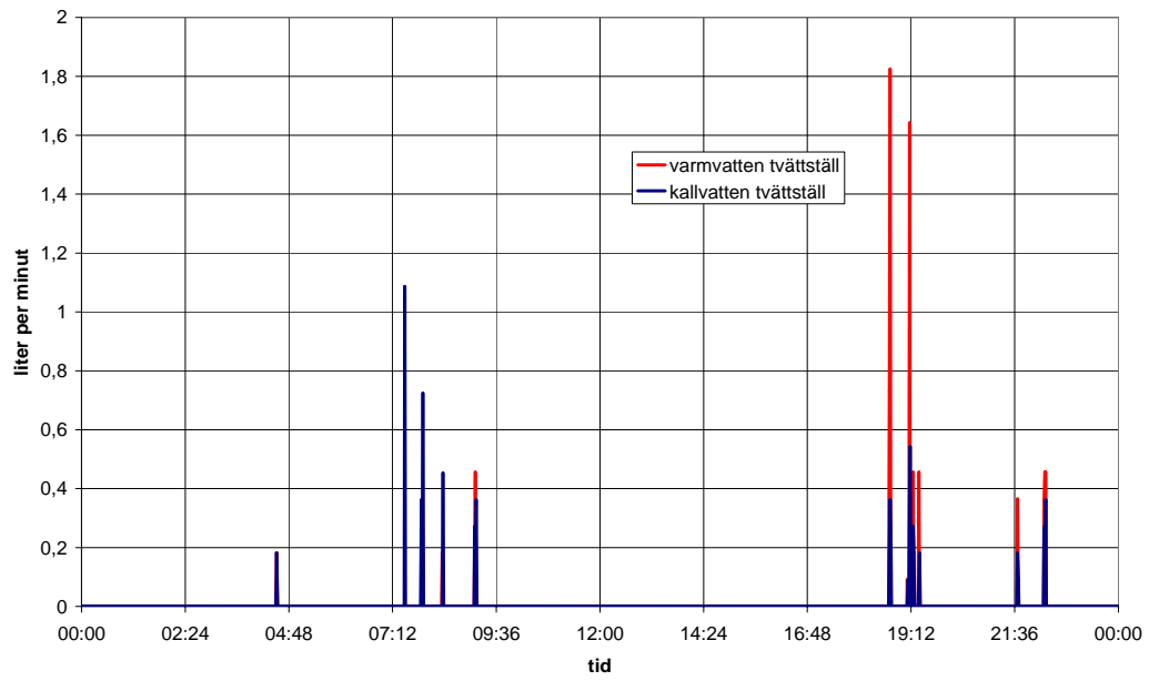
Figur C.6 Varm- och kallvattenanvändning i tvättställe under ett dygn i hushåll A (singel i lägenhet)
