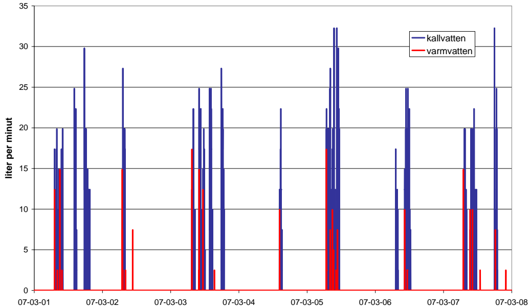
Figur 5.23 Vattenanvändning i tvättstuga A under en vecka
