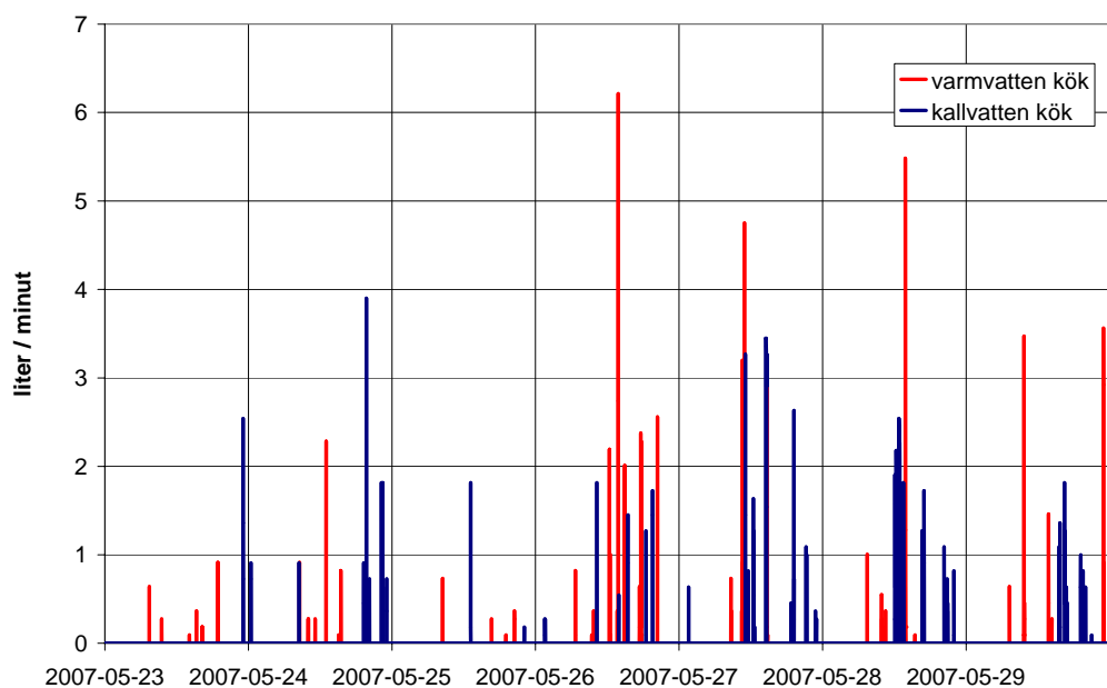
Figur 5.9 Varm- och kallvattenanvändning i kök under en vecka i hushåll E (singel i villa)
