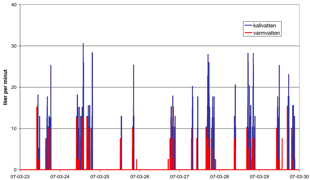
Figur 5.24 Vattenanvändning i tvättstuga C under en vecka
